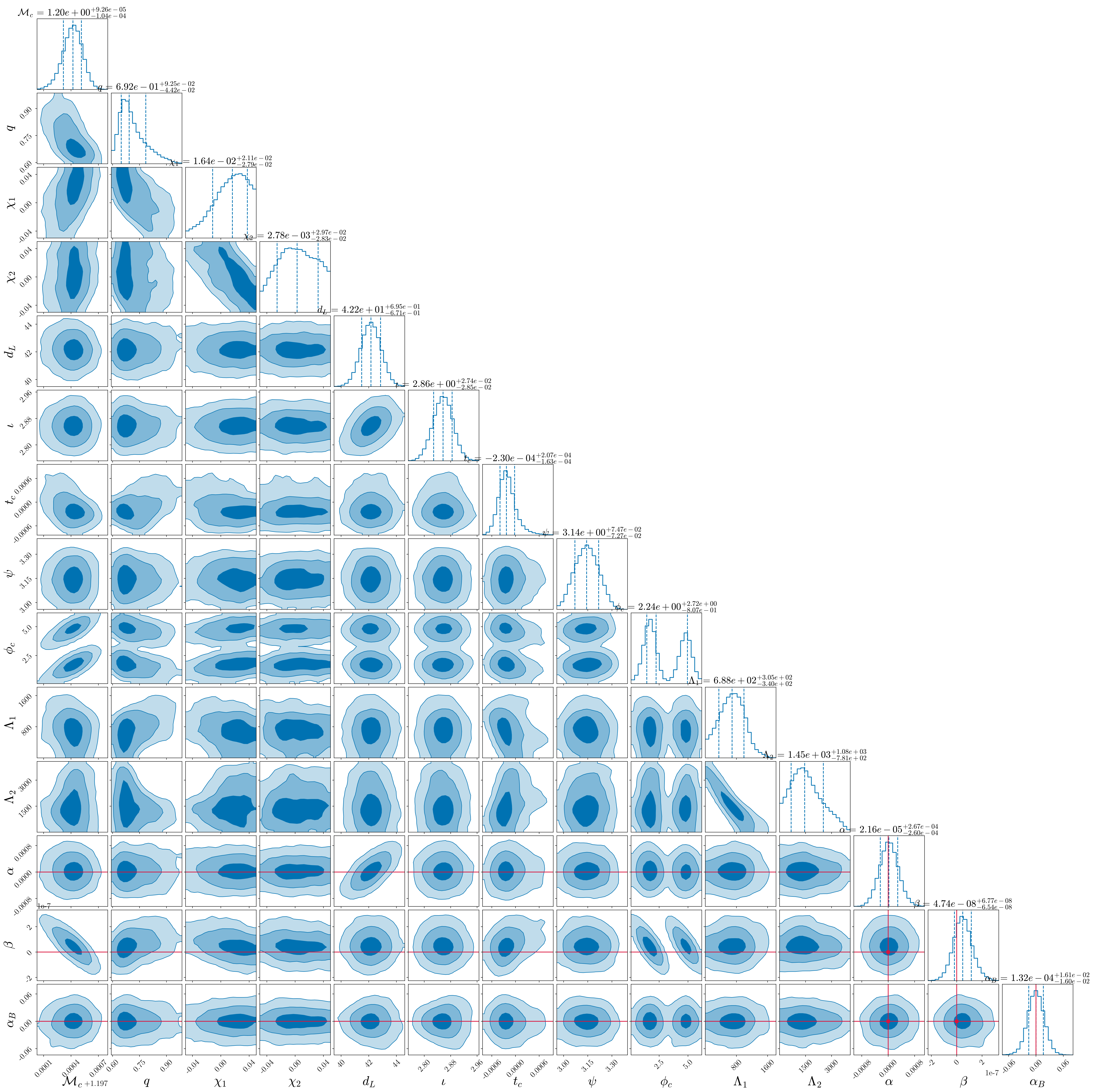
O5 HLV -- All Parameters (GW170817-like)
