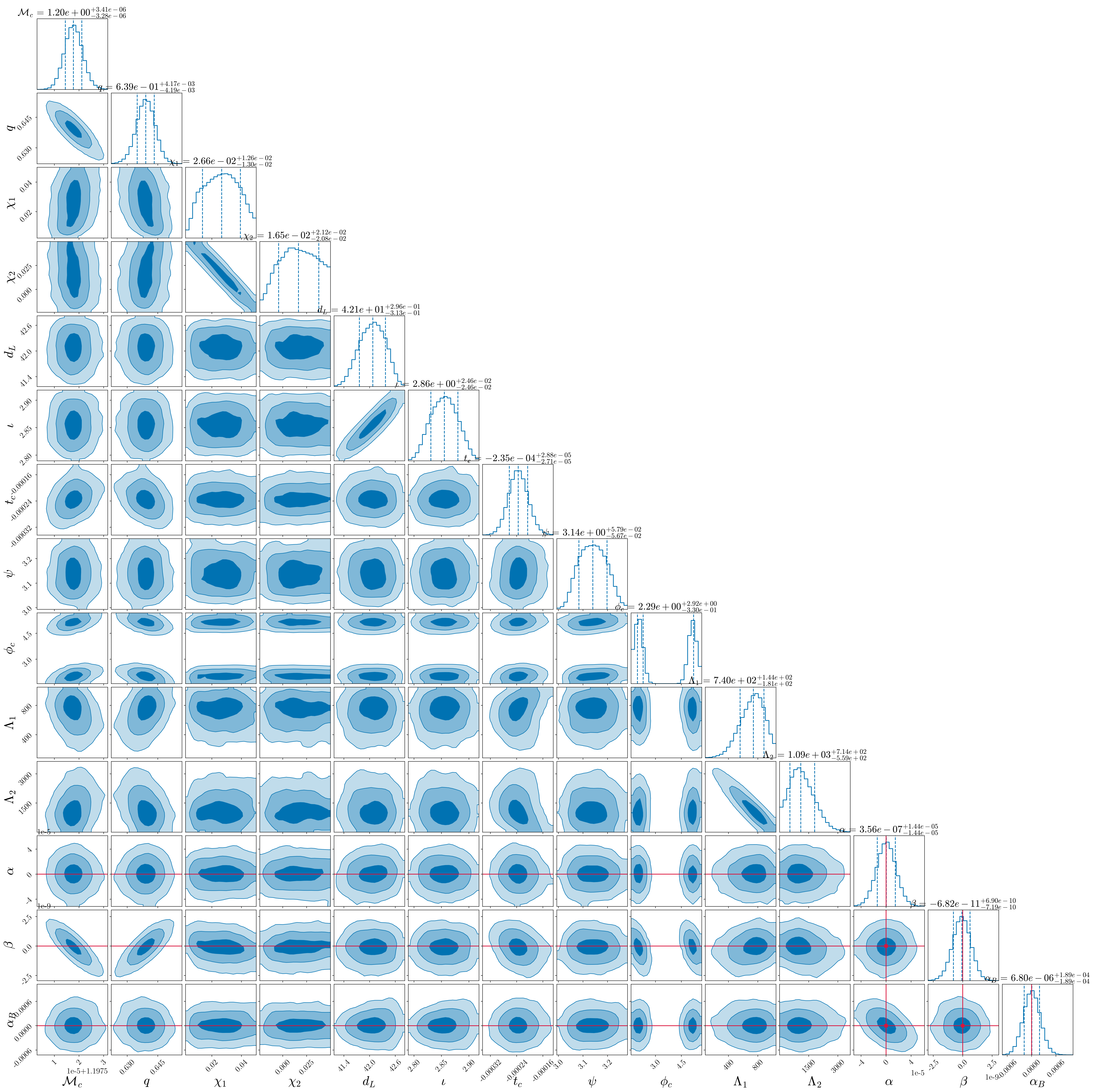
ETAΔ -- All Parameters (representative BNS)
