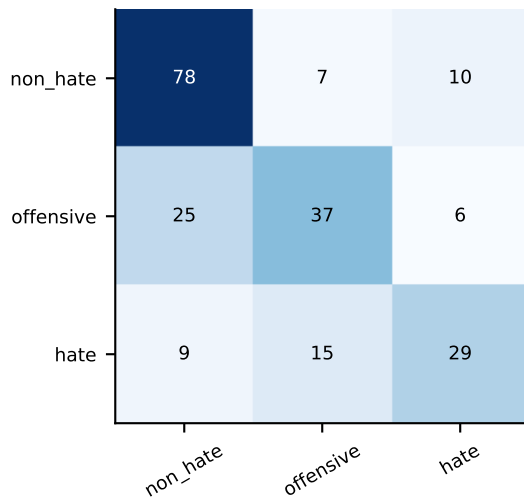
exp6_xlmr F1=0.431
