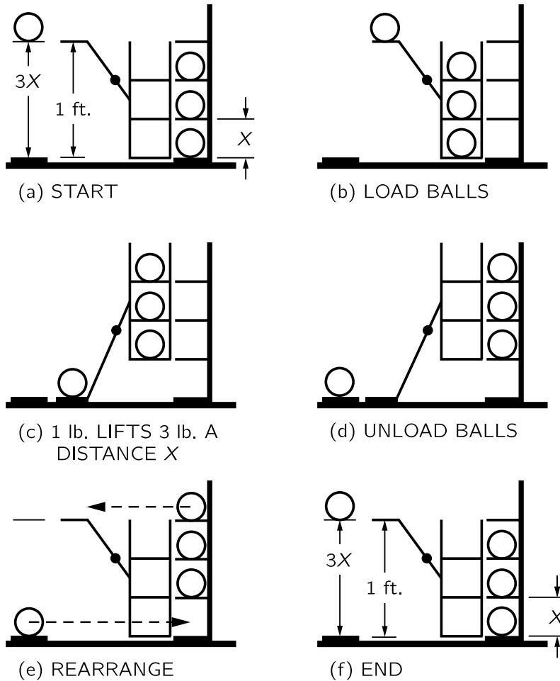
Fig. 4-2. A reversible machine.
