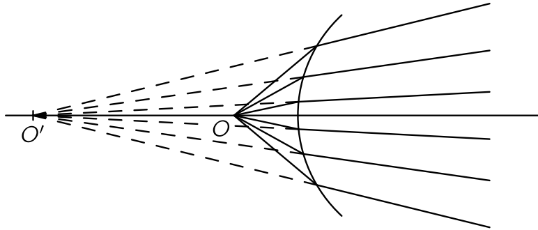
Fig. 27-3. A virtual image.
