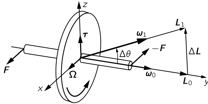
Fig. 20-2. A gyroscope.
