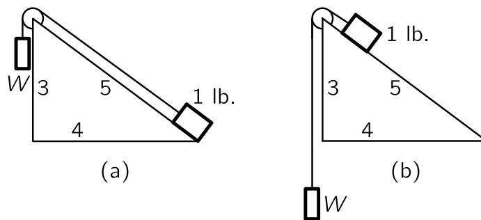
Fig. 4-3. Inclined plane.
