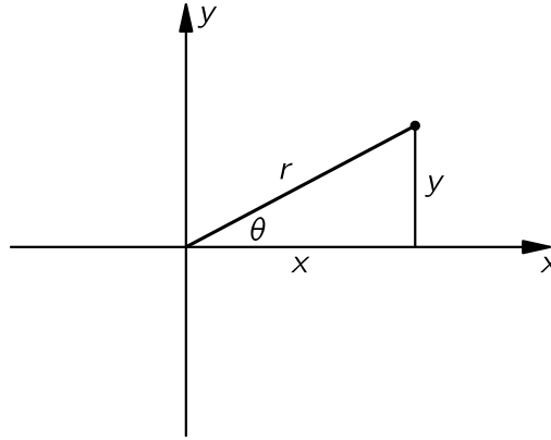
Fig. 22-2. x + iy = re^{i\theta} .
