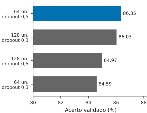
Figura 6 Ablation do LSTM, quatro variantes de unidades recorrentes e dropout , avaliadas por GroupKFold contra a decisão validada.
