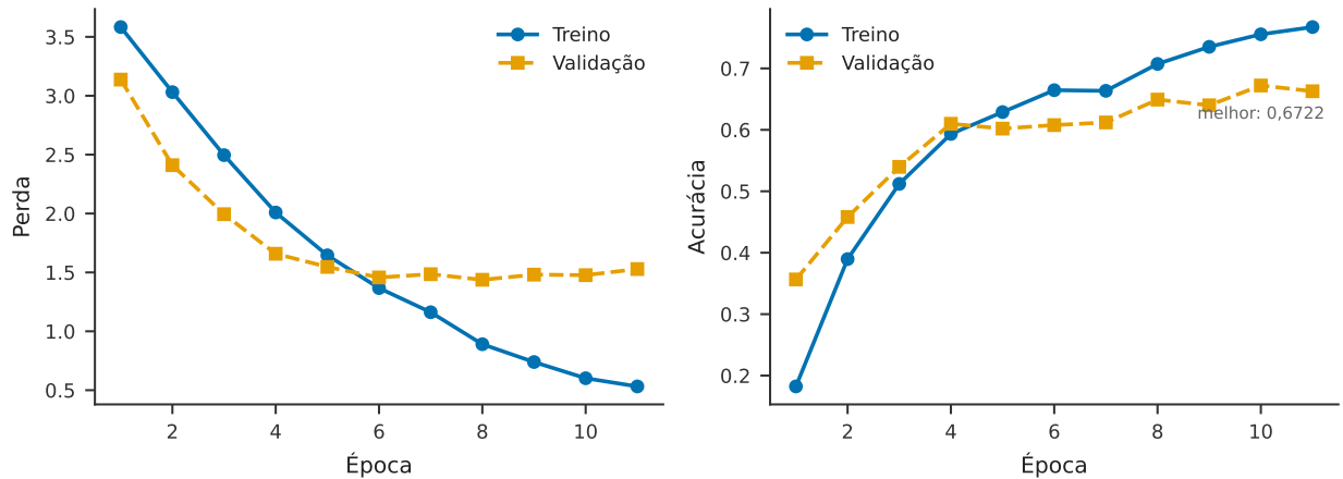
Figura 5 Curva de aprendizado do LSTM por época, perda e acurácia em treino e validação.
