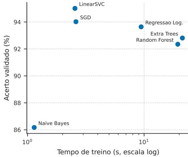
Figura 4 Trade-off entre acerto validado e tempo de treino, modelos clássicos.
