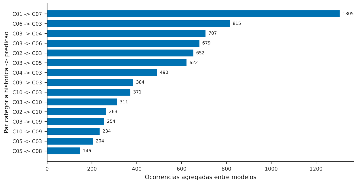
Figura 3 Quinze pares de categorias com maior confusão recíproca, agregados entre modelos. Os códigos do eixo vertical são descritos na Tabela Suplementar S2.
