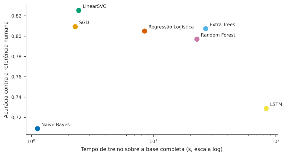
Figura 2: Trade-off entre acurácia e tempo de treino, modelos clássicos.
