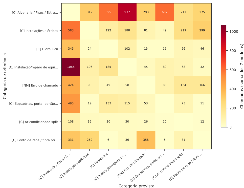
Figura 5: Recorte da matriz de confusão sobre as oito categorias mais envolvidas em troca recíproca, com contagens agregadas entre modelos.
