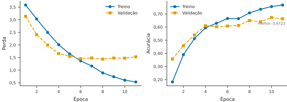
Figura 6: Curva de aprendizado do LSTM por época, perda e acurácia em treino e validação.
