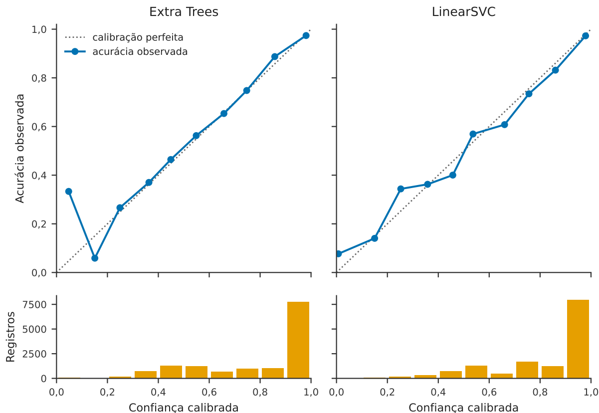
Figura 3: Curva de confiabilidade do Extra Trees e do LinearSVC após calibração isotônica, com confiança média e acurácia observada por faixa.
