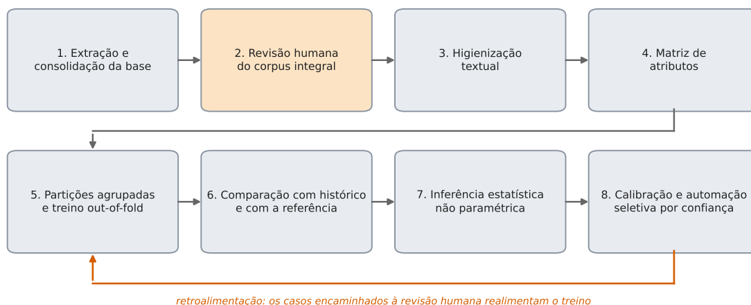
Figura 1: Pipeline de governança preditiva, do fluxo de extração da base à retroalimentação por validação humana.
