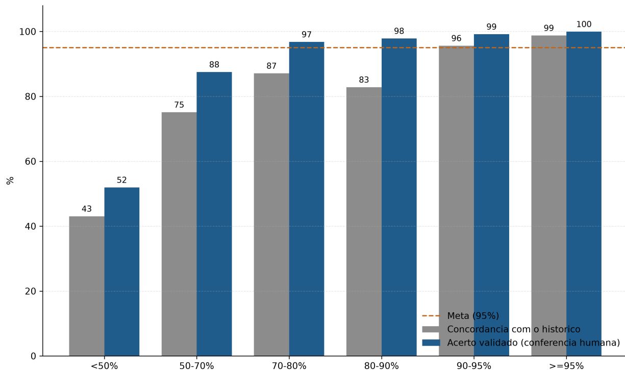
Figura 2: Figura 2 — Confiança bruta × concordância com o histórico × acerto validado, por faixa de confiança (executor oficial, Etapa 1).
