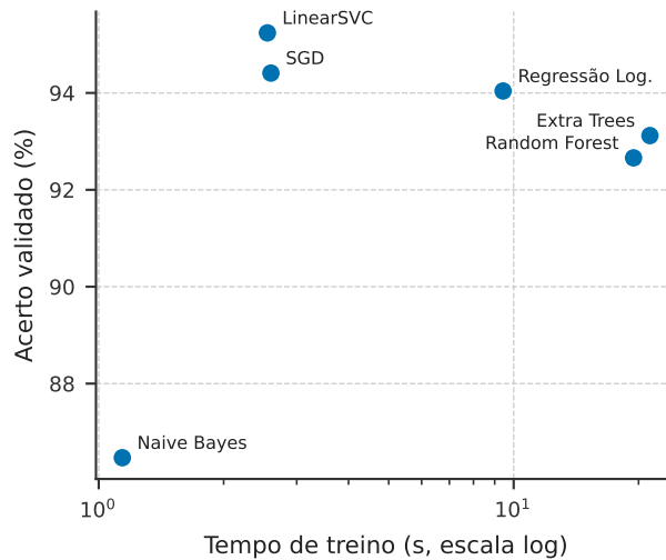
Figura 6: Trade-off entre acerto validado e tempo de treino, modelos clássicos.
