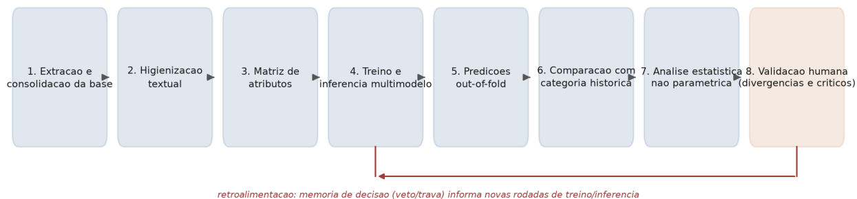
Figura 1: Pipeline de governança preditiva: fluxo metodológico completo, da extração da base à retroalimentação por validação humana.
