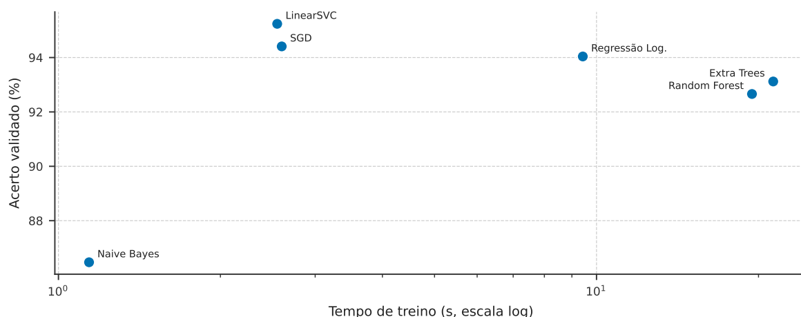
Figura 6: Trade-off entre acerto validado e tempo de treino, modelos clássicos.
