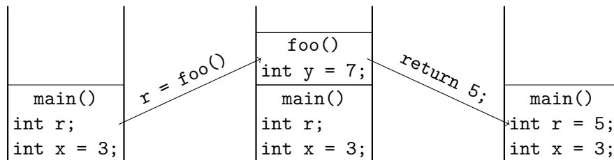
FIGURE 1 – Évolution de la pile lors d'appels et retours de fonction.
