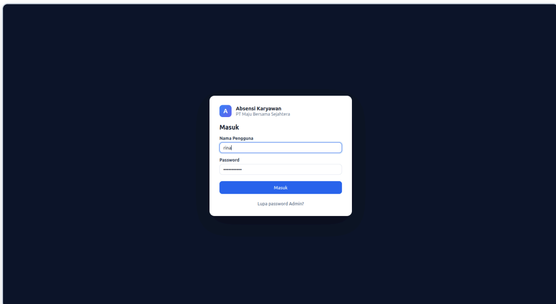
Gambar 2.3 — Layer masuk
