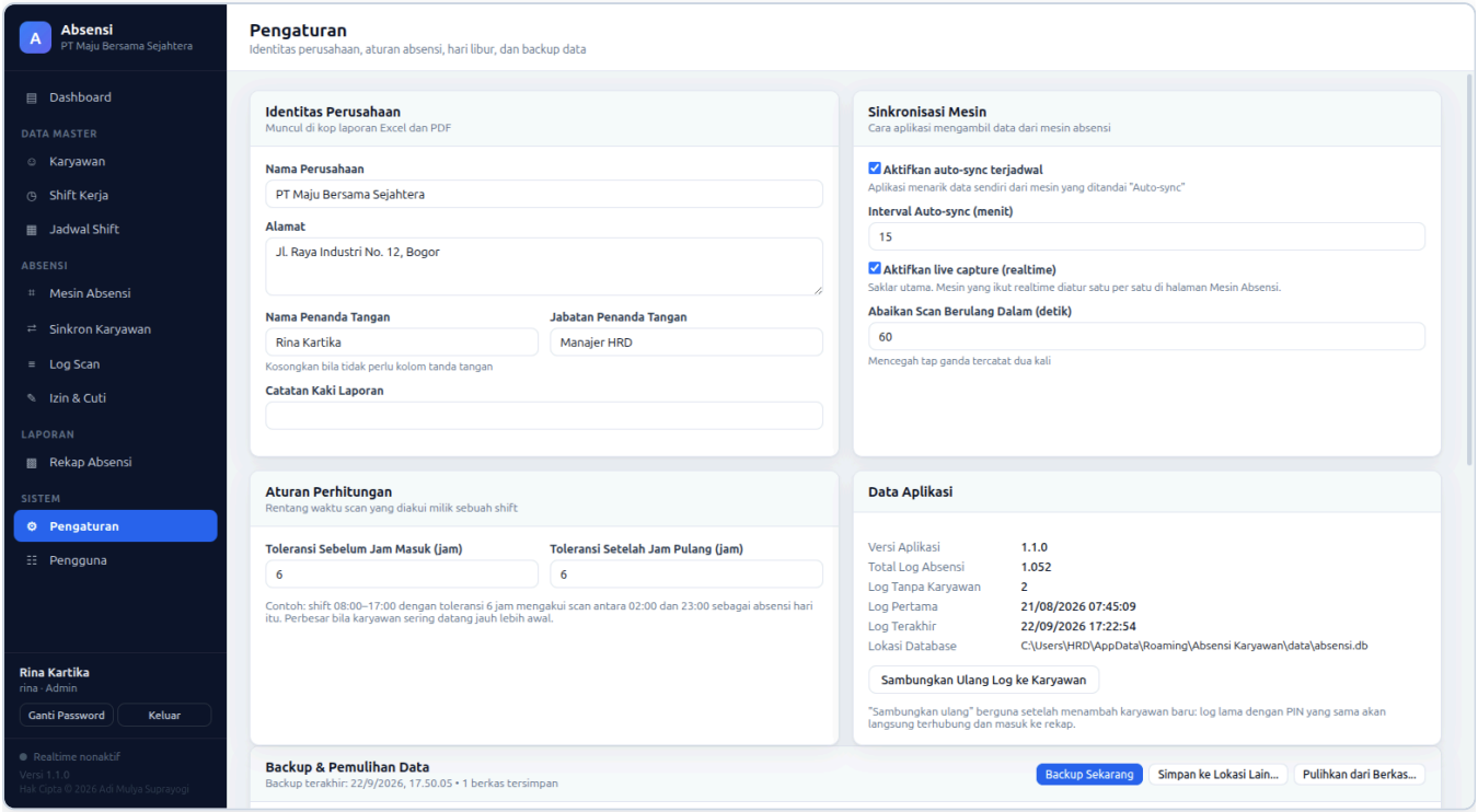
Gambar 12.1 — Pengaturan
