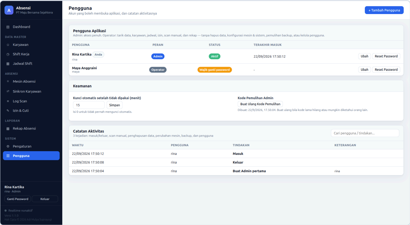
Gambar 13.1 — Halaman Pengguna
