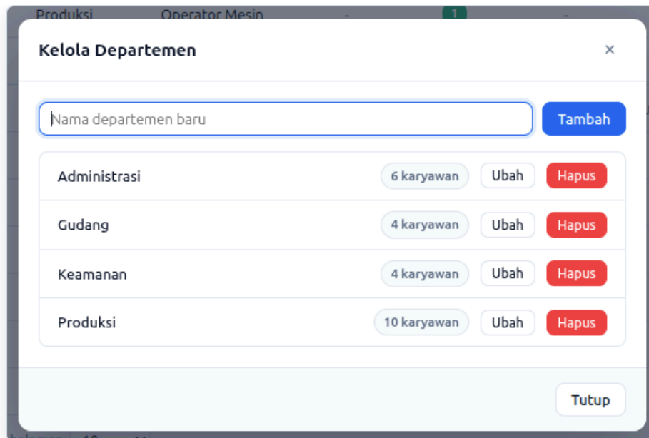
Gambar 5.7 — Kelola departemen
