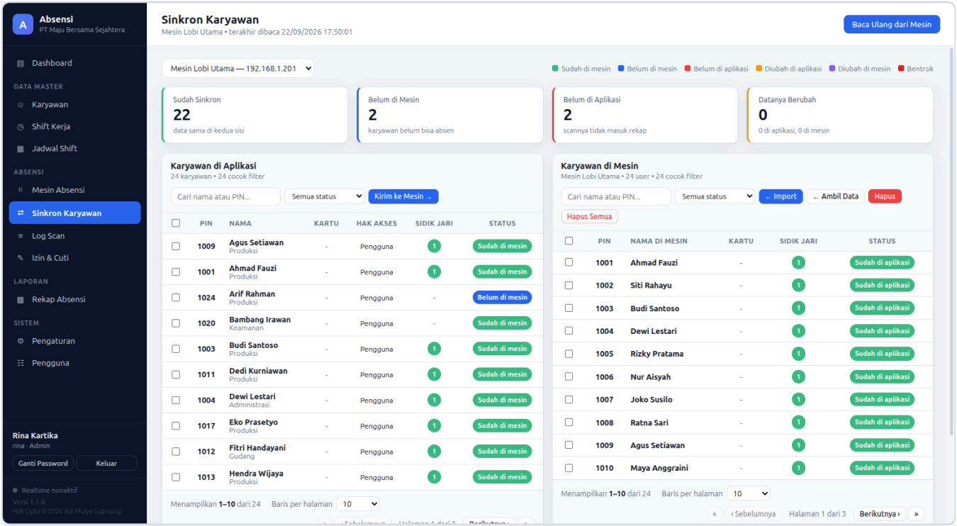
Gambar 6.1 — Sinkron Karyawan
