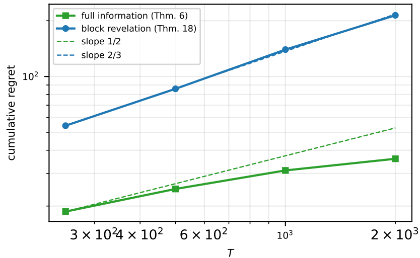
(d) n = 10 : regret growth, \sqrt{T} versus T^{2/3}
