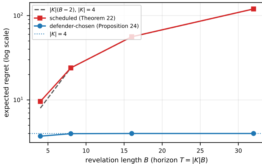
(d) same N = |K| reports: chosen times vs. fixed times
