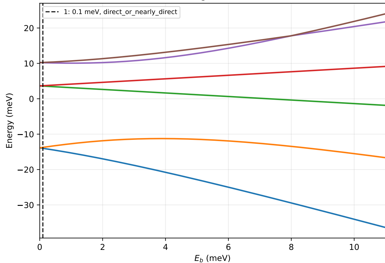
(a) Eigenvalues
