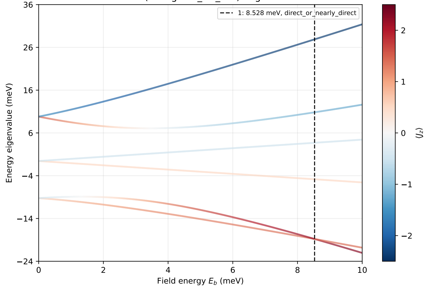
CeRhGe3 (tetragonal_D4_like): eigenvalues
