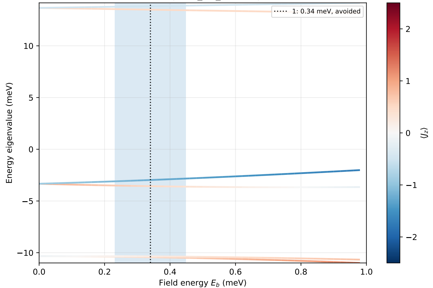
CeRhIn5 (tetragonal_D4_like): eigenvalues
