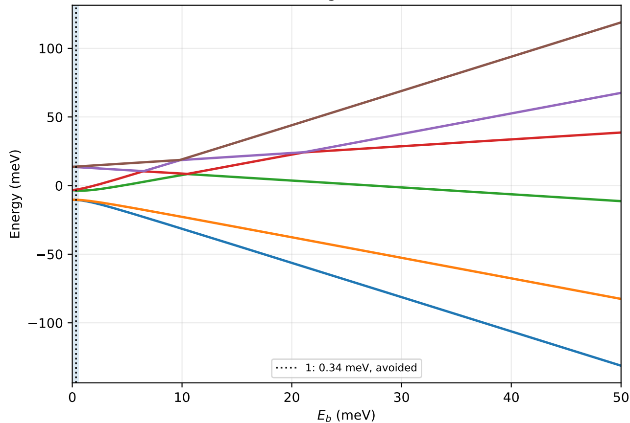
(a) Eigenvalues
