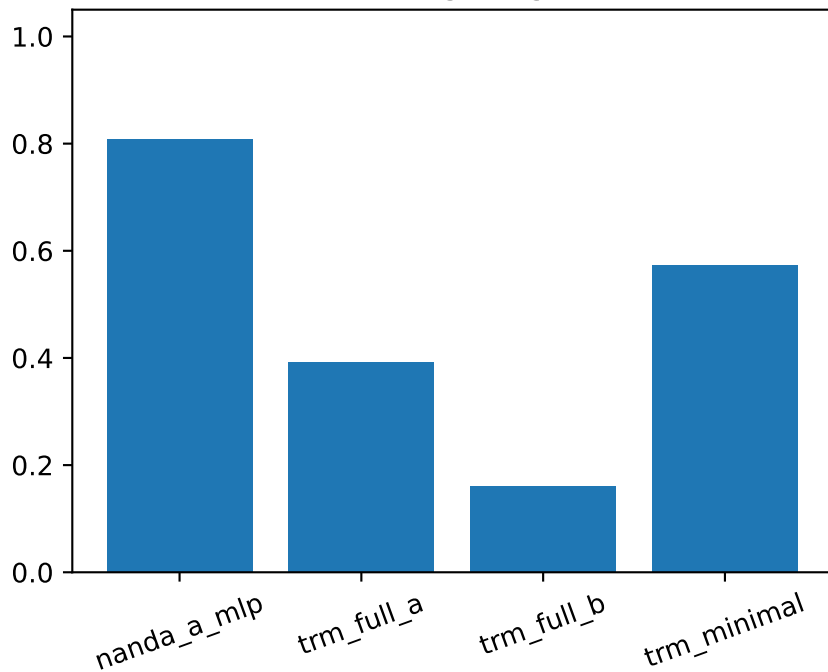
Faithful logit trig-FVE
