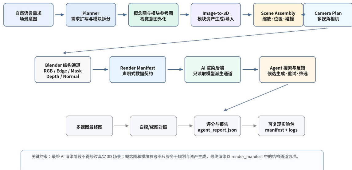
图 1 Harmonize3D 从自然语言到多视图成图的可审计闭环架构。
