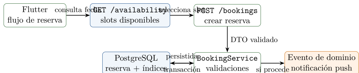
Figura 3.3: Flujo de creación de reserva y validación de disponibilidad
