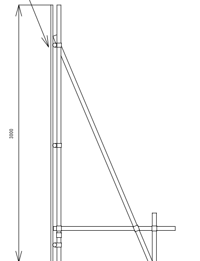
万能板仮囲い詳細図
