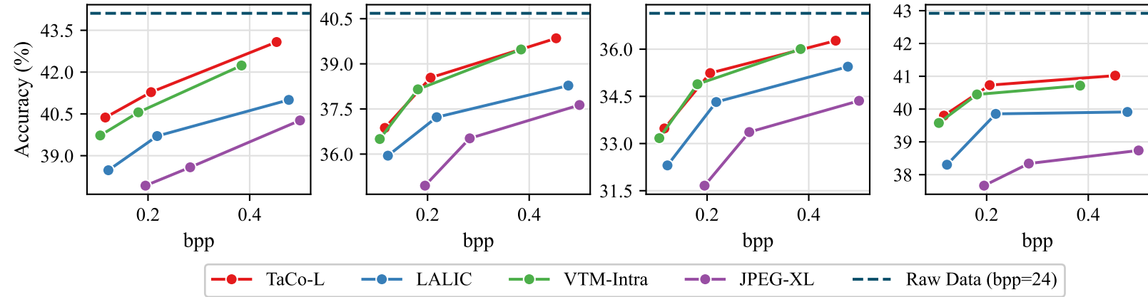
SVM
