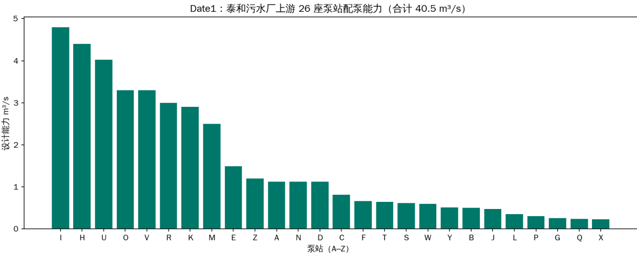
图 1-1 Date1：泰和污水厂上游 26 座泵站配泵能力 (合计约 40.5 m³/s)
