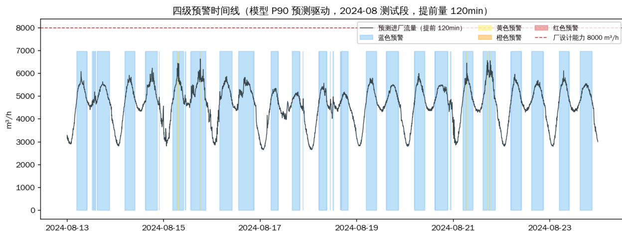
图 5-1 四级预警时间线（模型 P90 预测驱动，2024-08 测试段强降雨过程，提前量 120 min）
