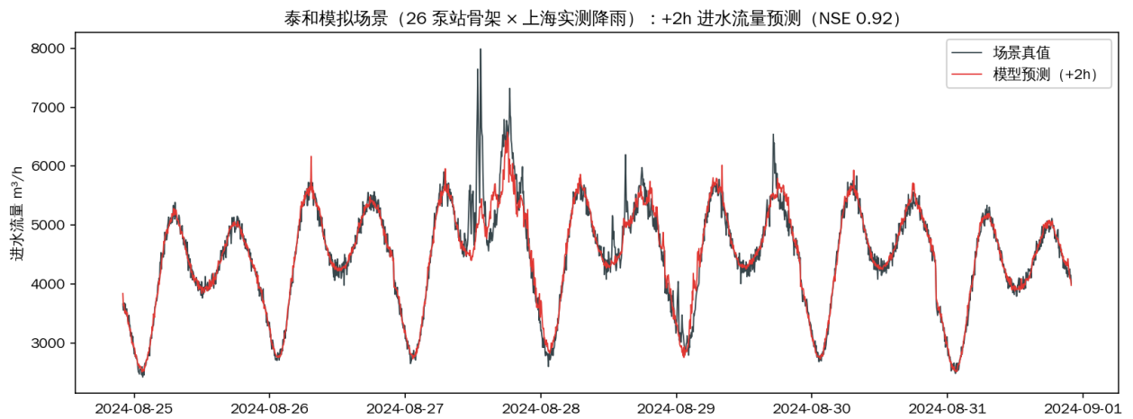
图 4-3 泰和模拟场景 +2h 进水流量预测 (测试集末 7 天)
