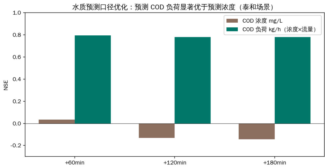
图 4-7 水质预测口径优化：COD 负荷显著优于浓度
