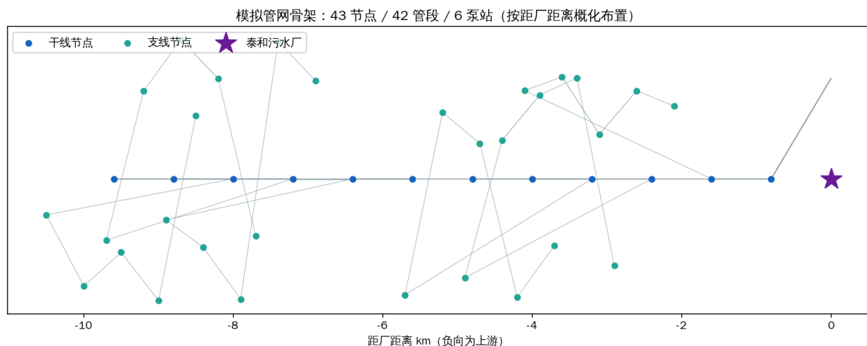
图 3-1 模拟管网骨架：43 节点 / 42 管段 / 6 泵站（按距厂距离概化布置）
