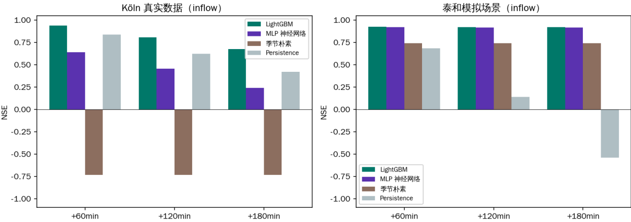
图 4-5 四模型 NSE 对比（左：Köln 真实数据；右：泰和模拟场景）
