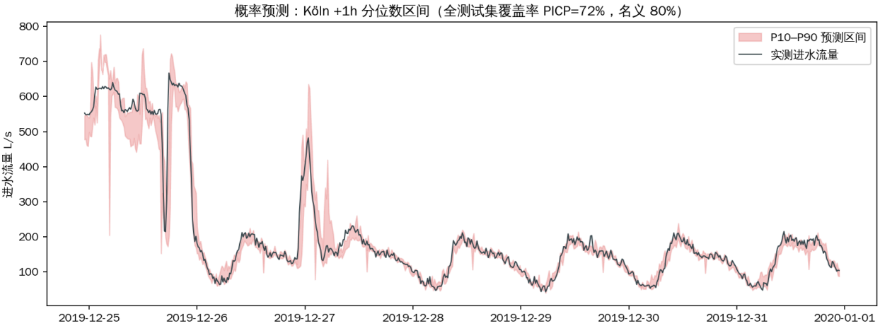
图 4-6 概率预测：Köln +1h P10–P90 分位数区间
