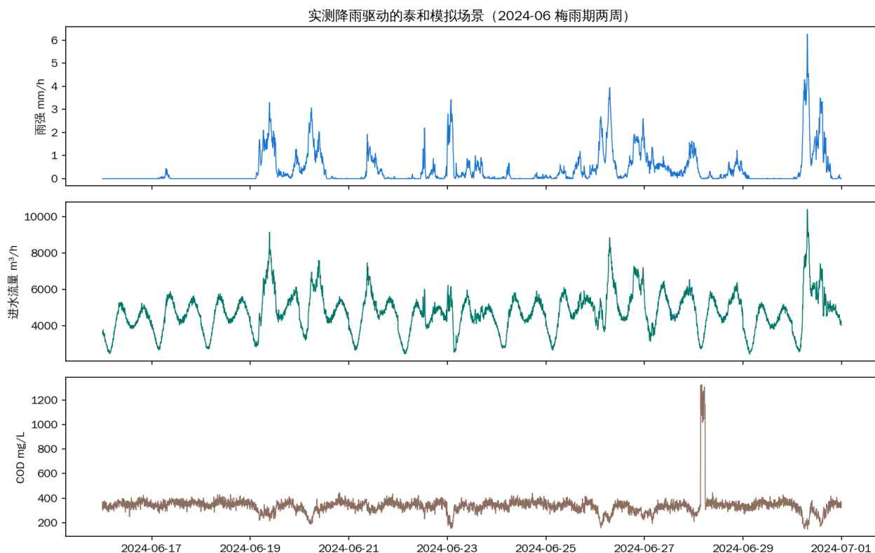
图 3-2 实测降雨驱动的泰和模拟场景（2024-06 梅雨期两周：雨强 → 进水流量 → COD）
