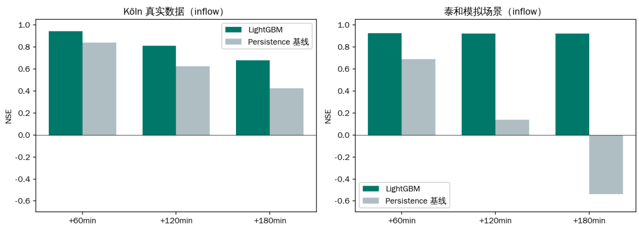
图 4-4 提前量—精度对比 : LightGBM vs persistence (左 : Köln 真实数据 ; 右 : 泰和模拟场景)
