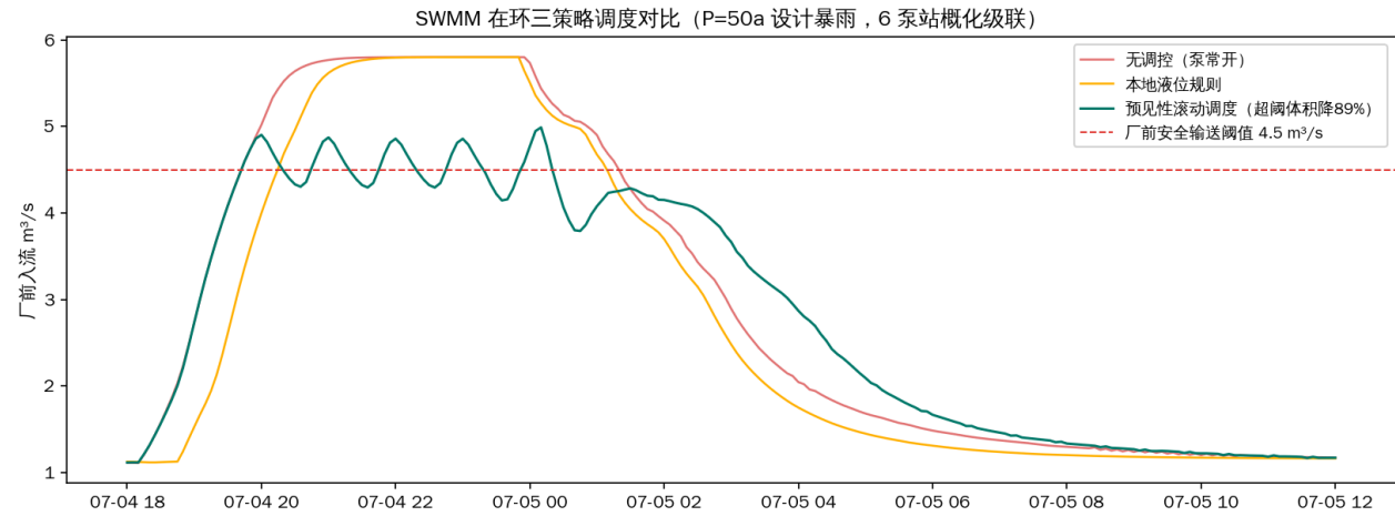
图 5-2 SWMM 在环调度对比：预见性滚动调度将厂前入流控制在安全阈值附近 (P=50a 设计暴雨)
