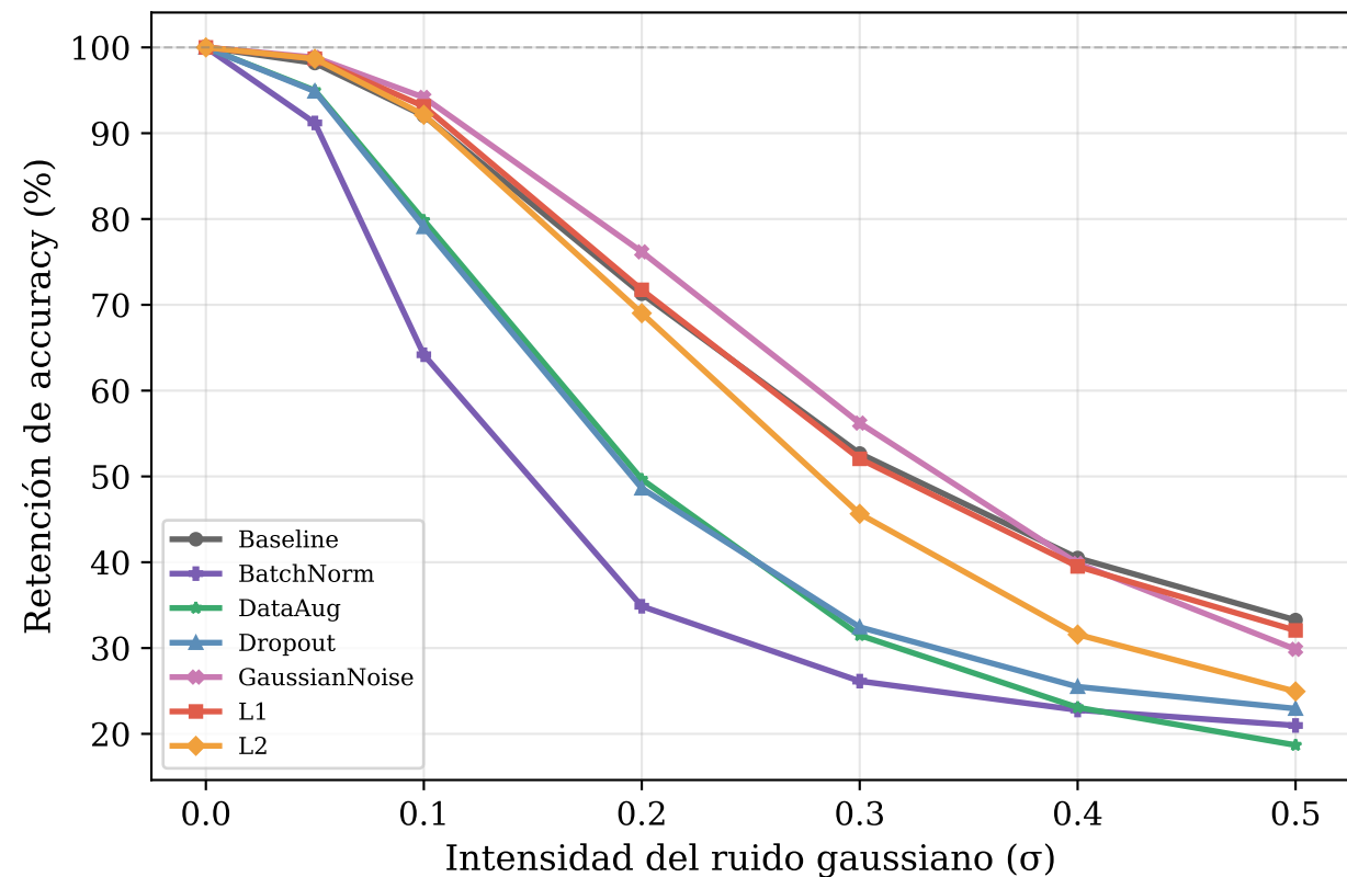
Retención relativa vs Ruido en datos
