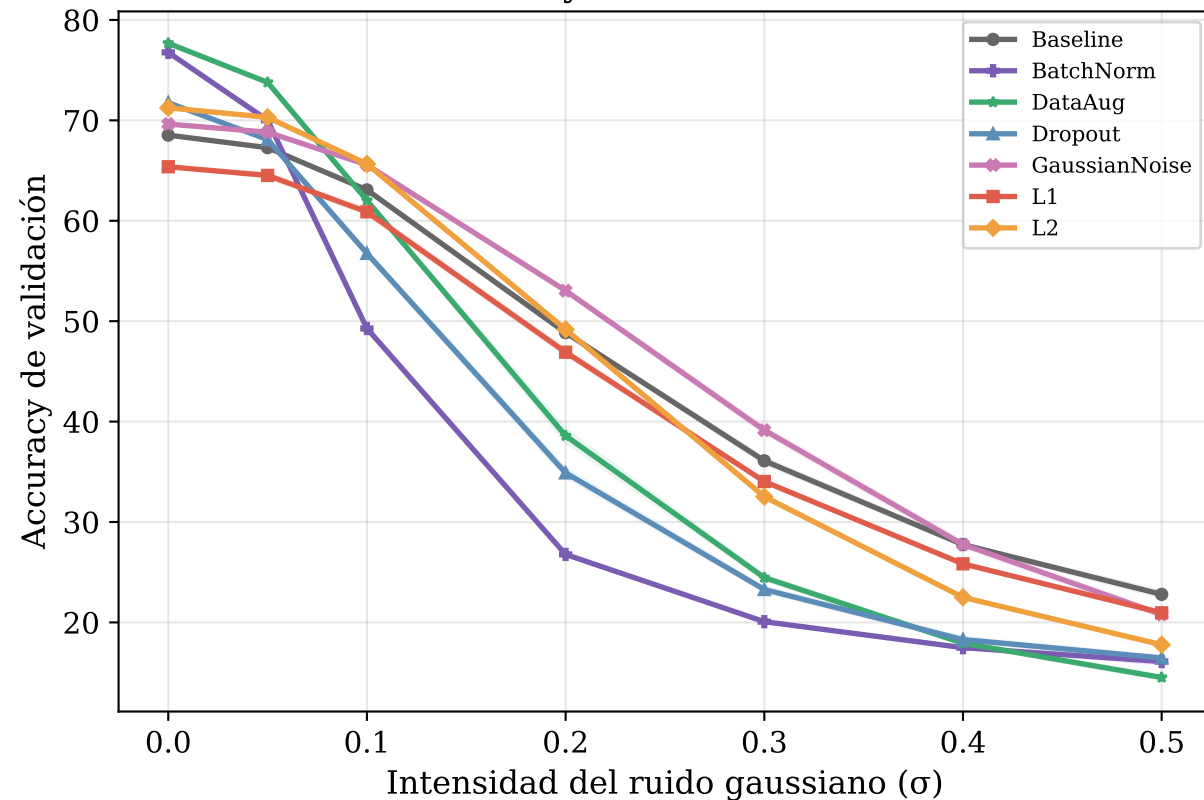
Accuracy vs Ruido en datos
