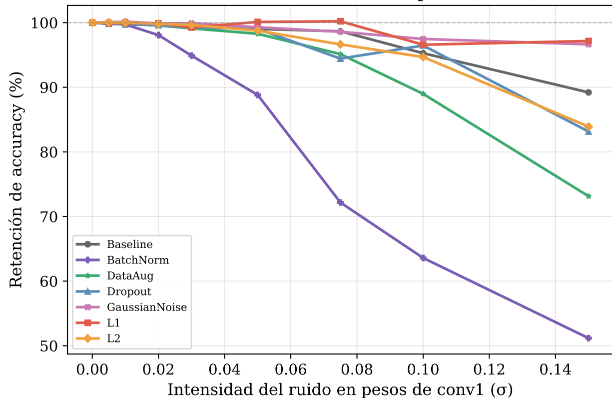
Retención relativa vs Ruido en pesos (conv1)
