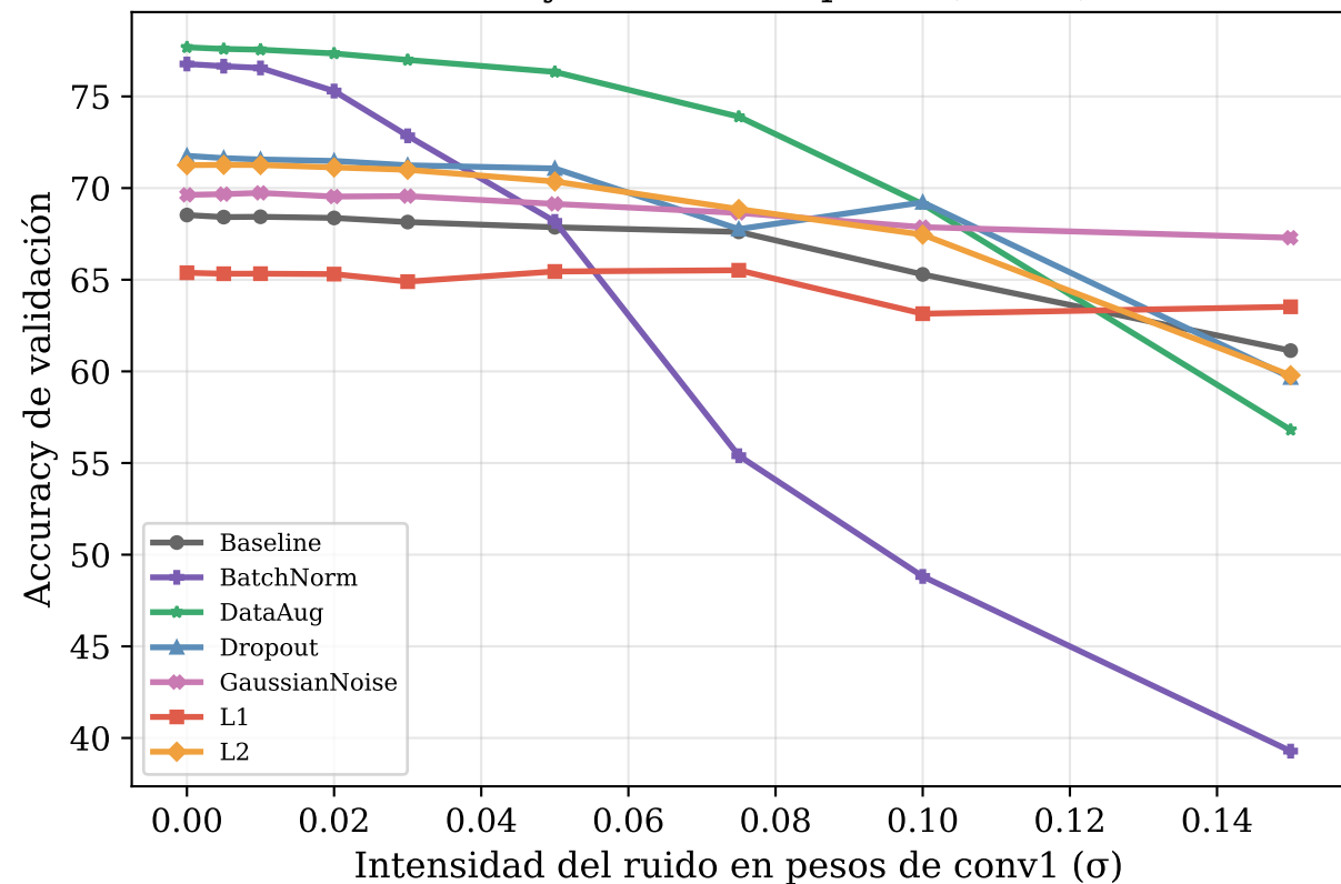
Accuracy vs Ruido en pesos (conv1)
