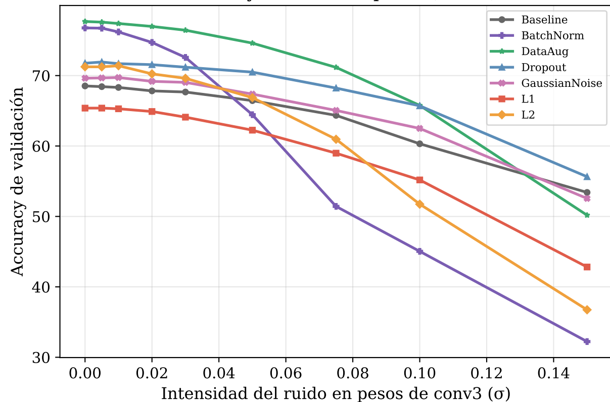
Accuracy vs Ruido en pesos (conv3)
