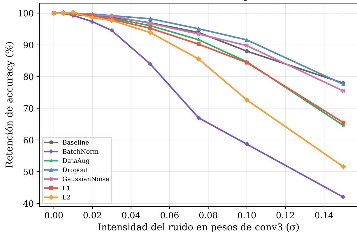
Retención relativa vs Ruido en pesos (conv3)
