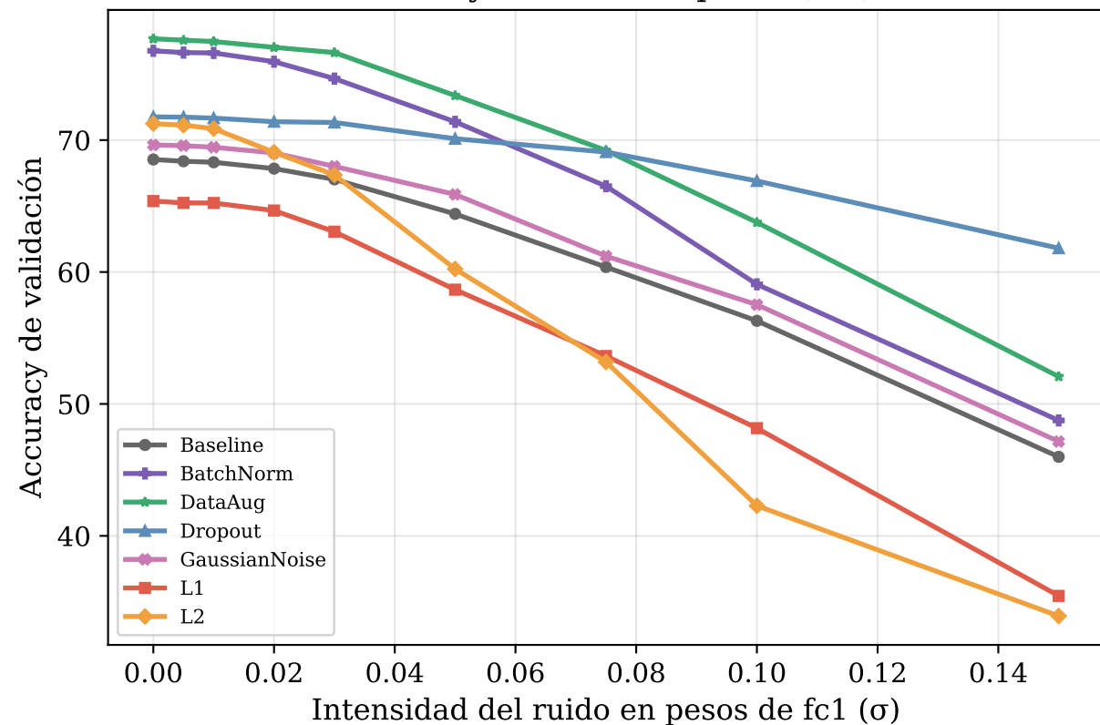
Accuracy vs Ruido en pesos (fc1)
