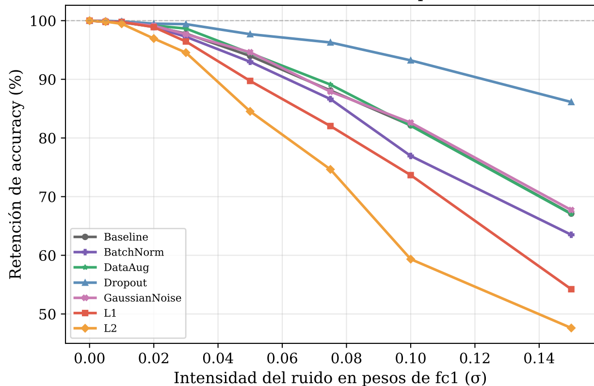
Retención relativa vs Ruido en pesos (fc1)
