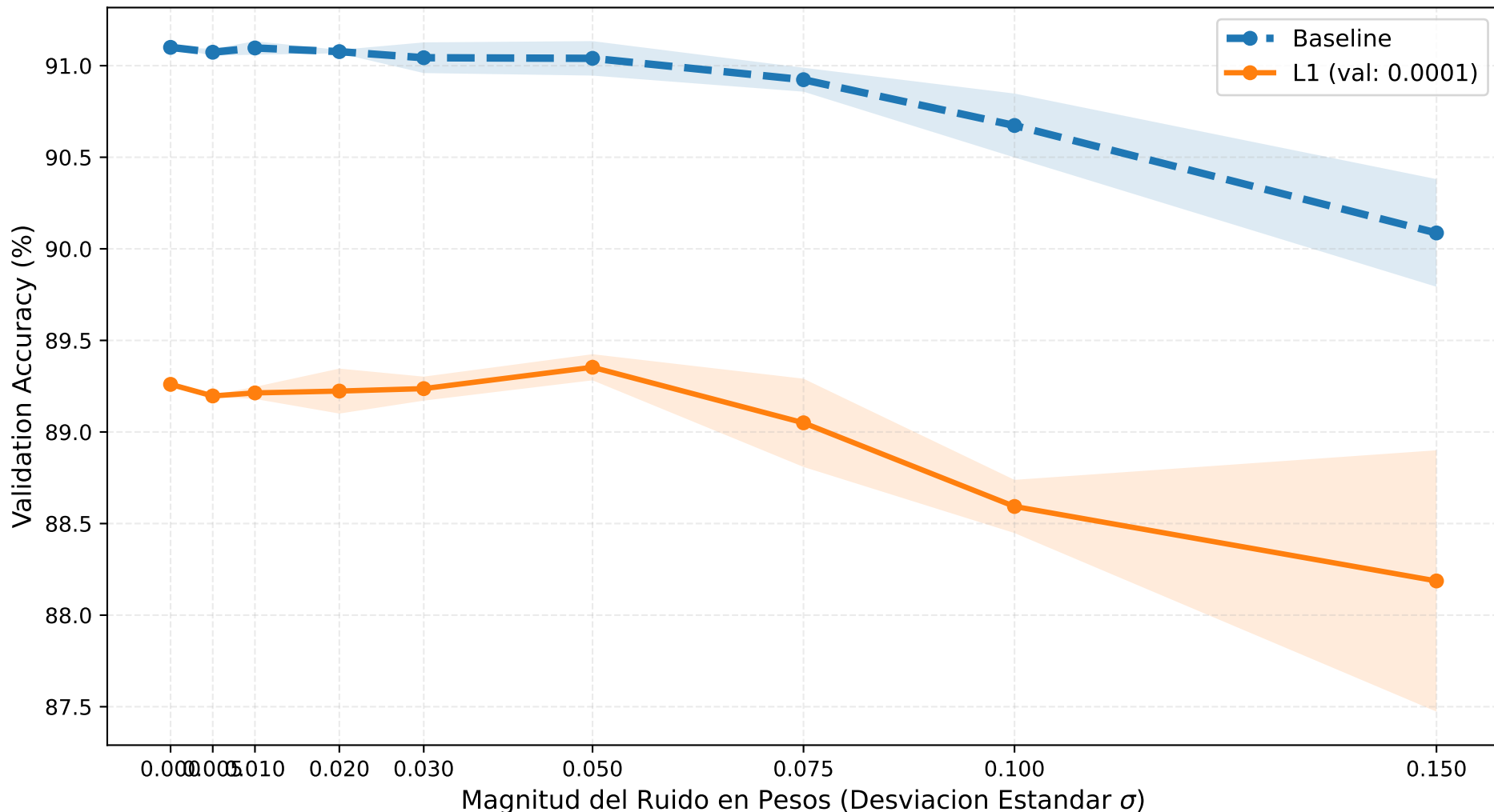
Robustez a la Perturbacion de Pesos (Flat Minima Test)
