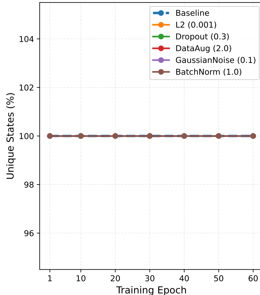
Capa: CONV1
