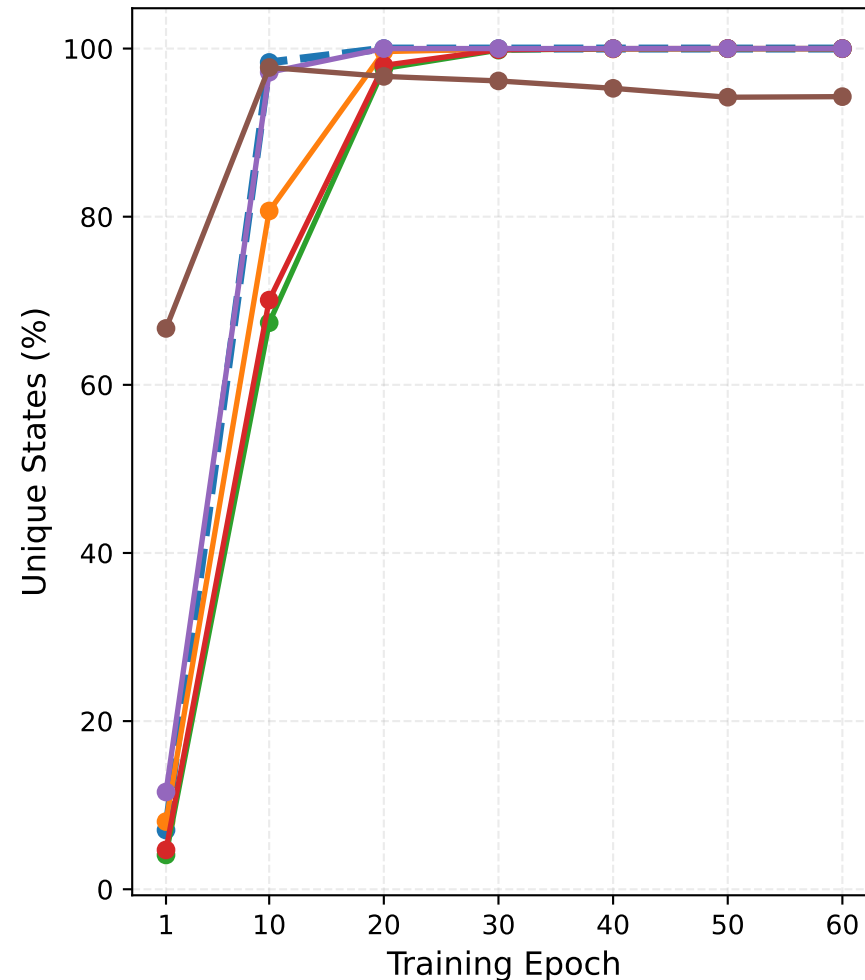
Capa: CONV3
