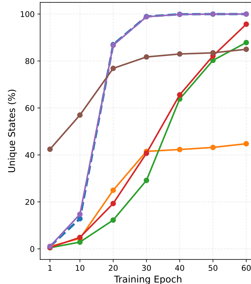
Capa: FC1
