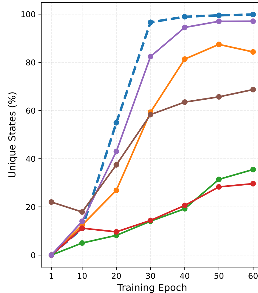
Capa: FC1
