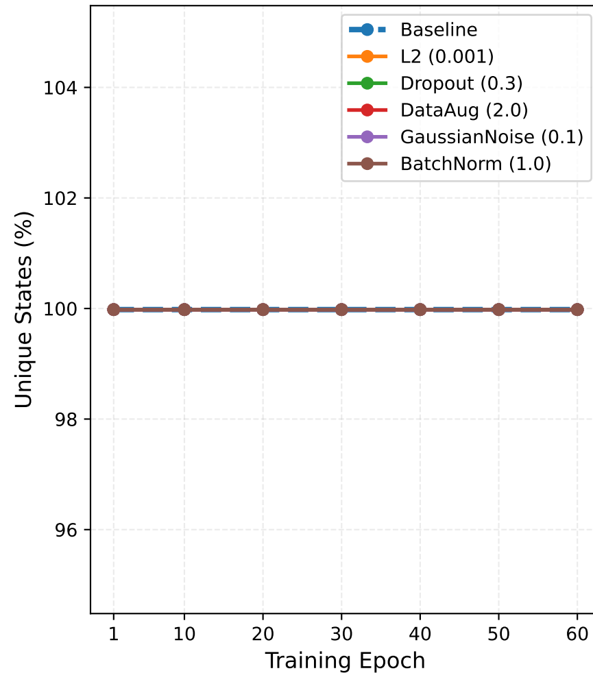
Capa: CONV1
