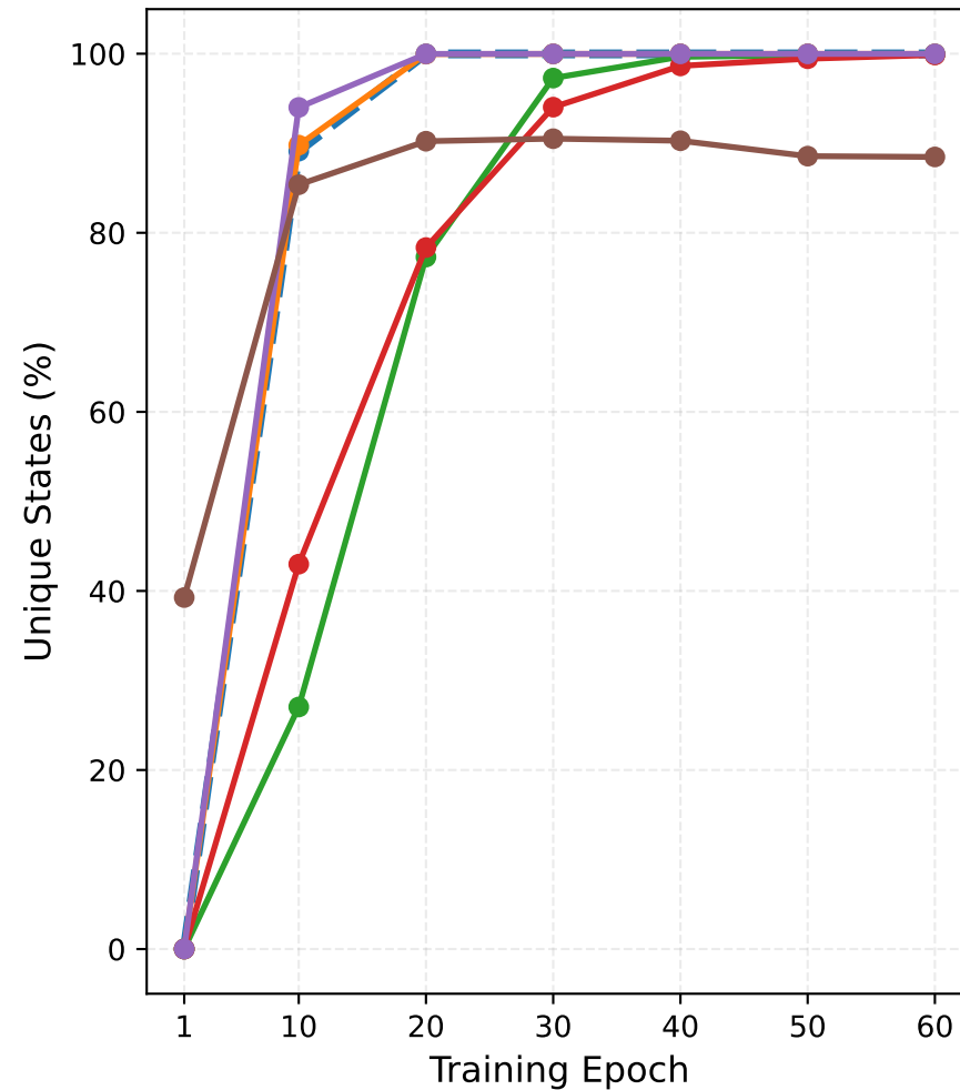
Capa: CONV3
