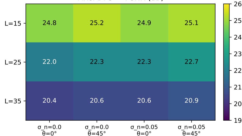
Pixel-DPS — PSNR (dB)
