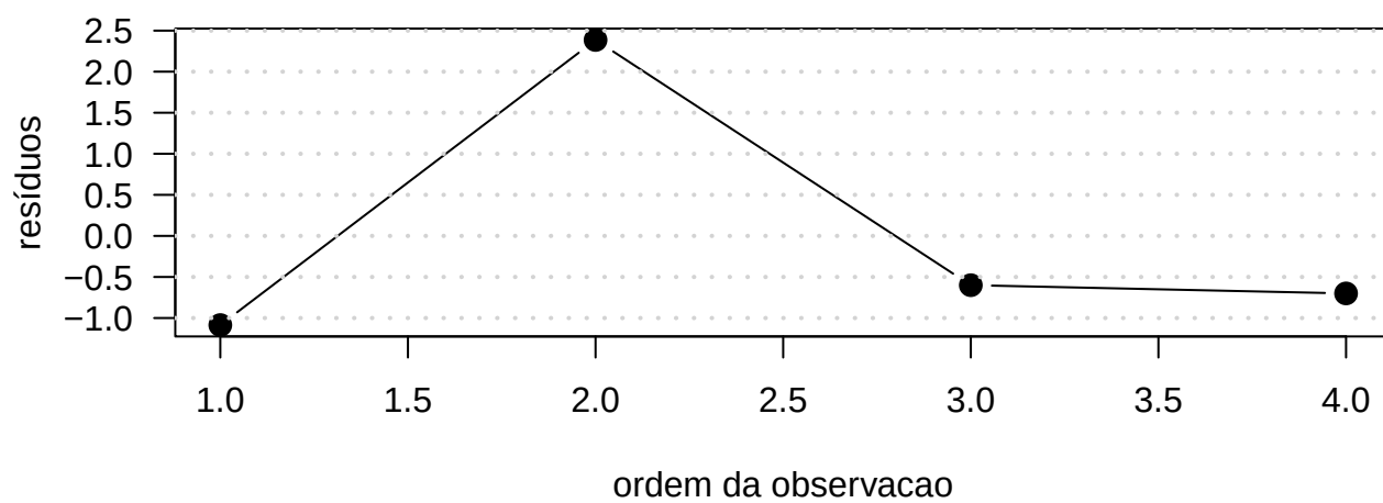
Figure 3: Resíduos do IMC da população feminina em função da ordem de observação.
