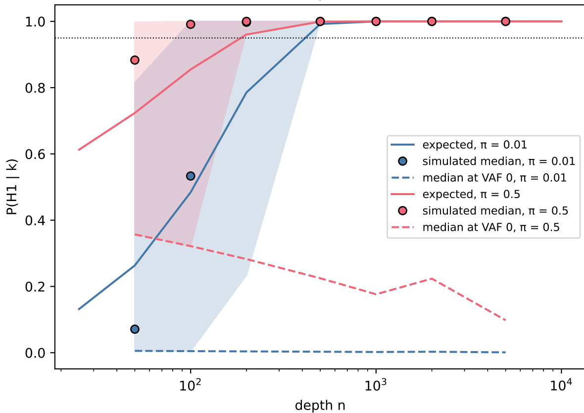
Posterior vs depth at VAF 0.02
