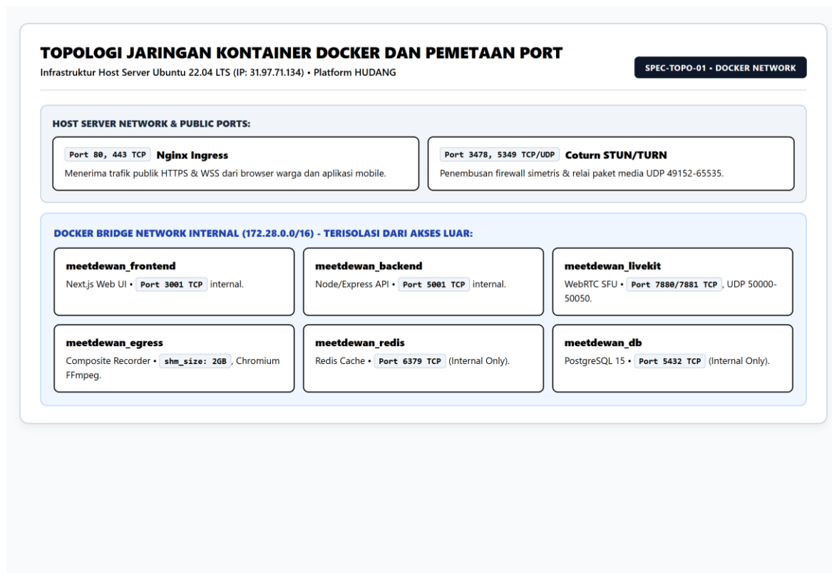
Gambar 2.2: Diagram Topologi Jaringan Kontainer Docker dan Pemetaan Port Host Server
