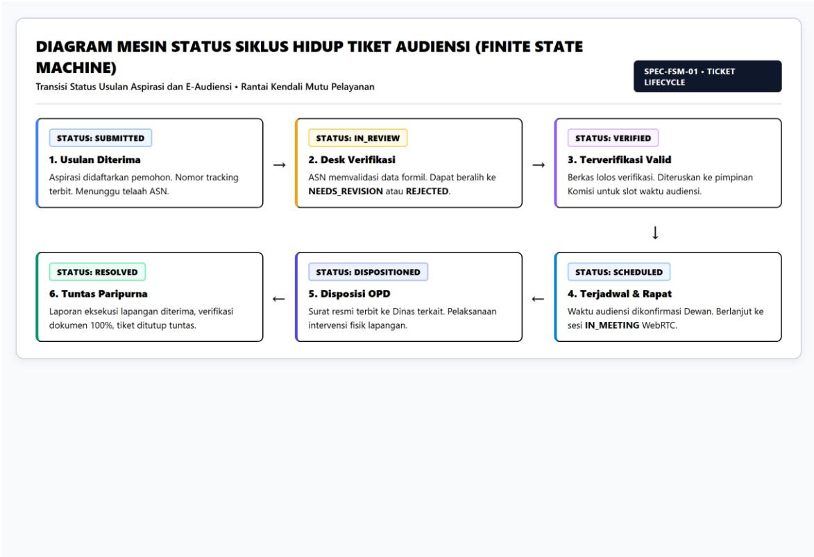
Gambar 5.2: Diagram Mesin Status Siklus Hidup Tiket Audiensi (Finite State Machine)
