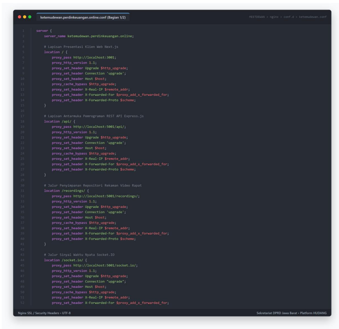
Gambar 2.4a: Cuplikan Konfigurasi Gateway Proksi Nginx (SSL, WAF & Security Headers)
