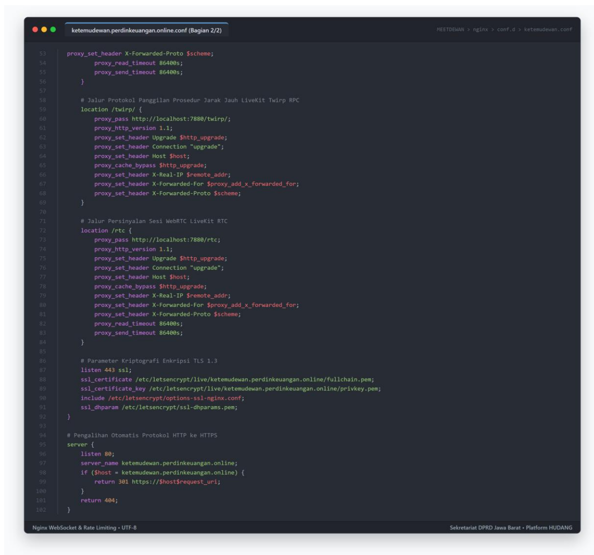
Gambar 2.4b: Cuplikan Konfigurasi Gateway Proksi Nginx (WebSocket, Media & Rate Limiting)
