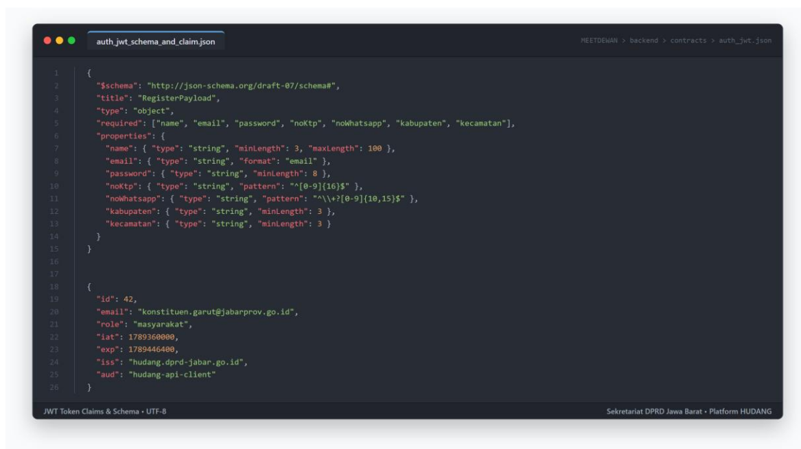
Gambar 3.7: Cuplikan Skema Endpoint Autentikasi dan Struktur Klaim Token JWT
