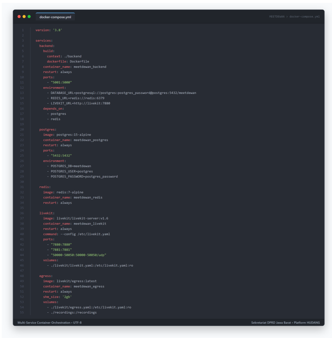
Gambar 4.3: Cuplikan Kode Sumber Orkestrasi Kontainer Sistem (docker-compose.yml)
