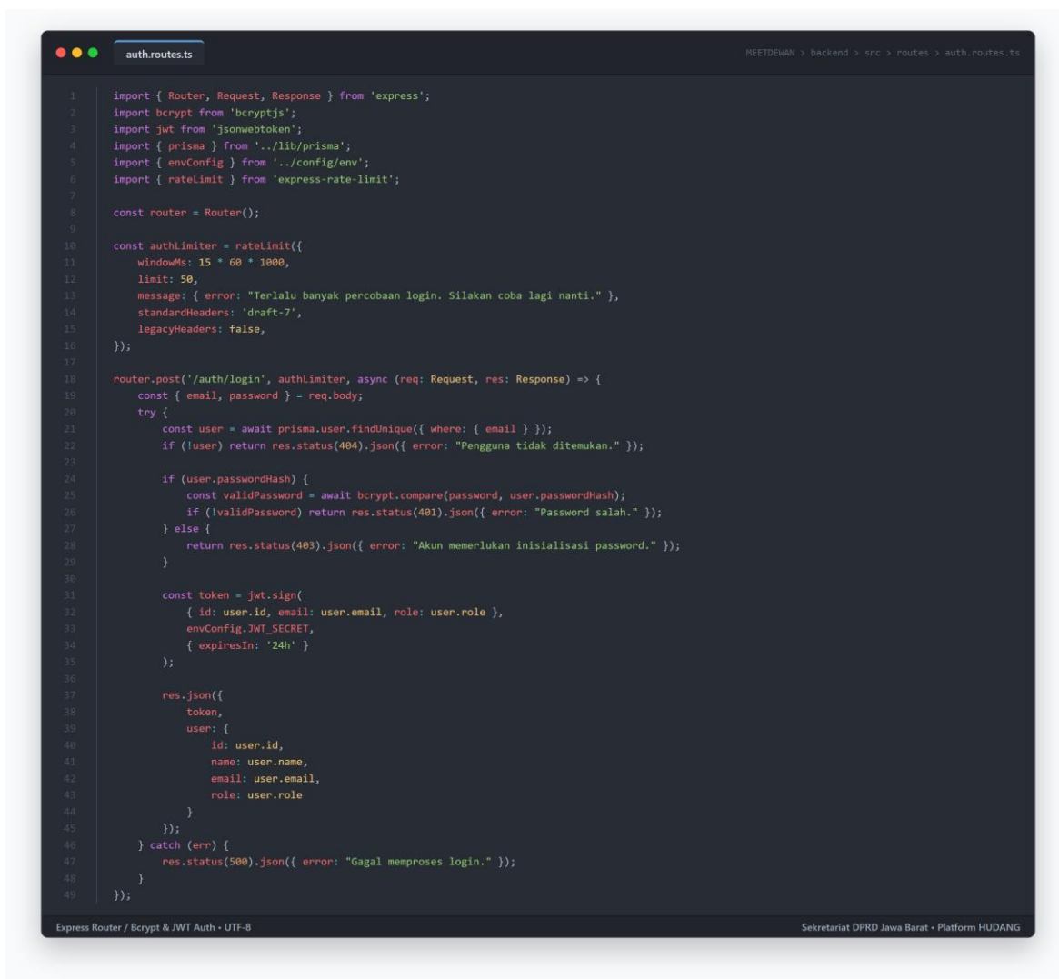
Gambar 4.5: Cuplikan Kode Sumber Otentikasi dan Pengamanan Akses API (auth.routes.ts)
