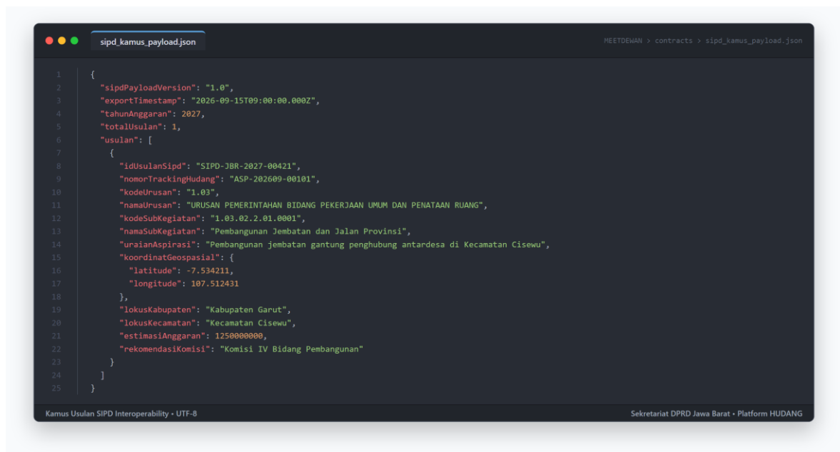
Gambar 3.9: Cuplikan Format Kamus Usulan Interoperabilitas SIPD Republik Indonesia
