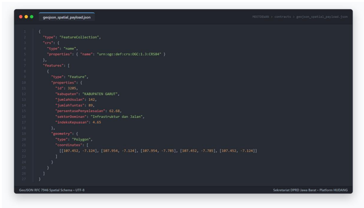
Gambar 3.10: Cuplikan Skema Spasial Tematik GeoJSON FeatureCollection (RFC 7946)
