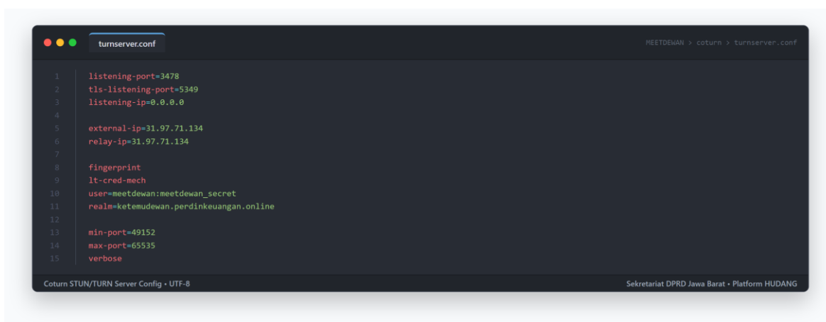
Gambar 2.6: Cuplikan Konfigurasi Server NAT Coturn STUN/TURN (turnserver.conf)
