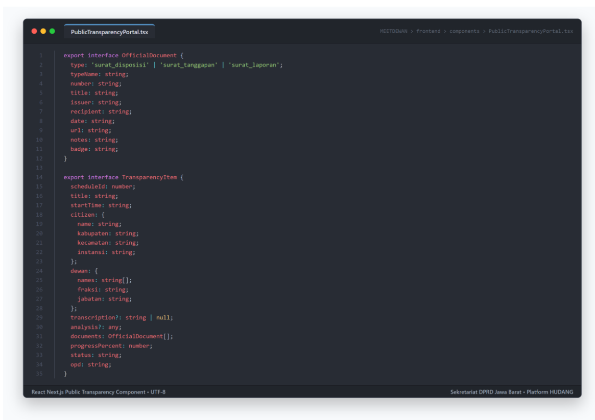
Gambar 4.8: Cuplikan Kode Sumber Antarmuka Keterbukaan Publik (PublicTransparencyPortal.tsx)
