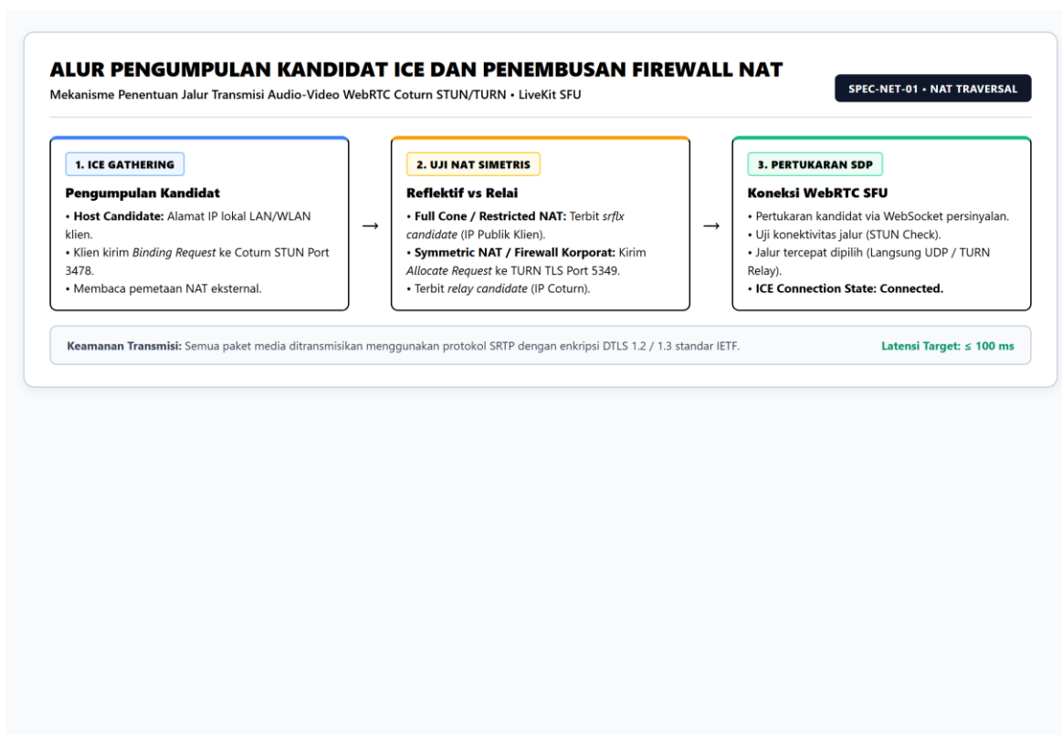
Gambar 2.3: Diagram Alur Pengumpulan Kandidat ICE dan Penembusan Firewall NAT Coturn STUN/TURN
