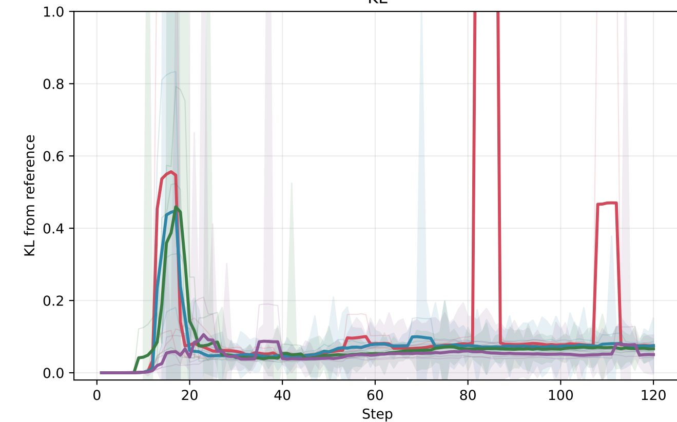
KL
