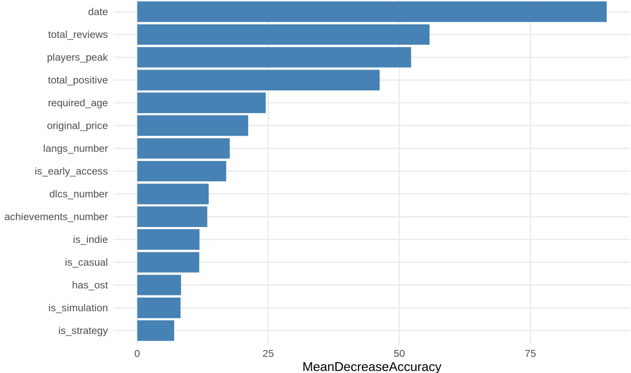
Figura 5: Variables más relevantes para el modelo Random Forest
