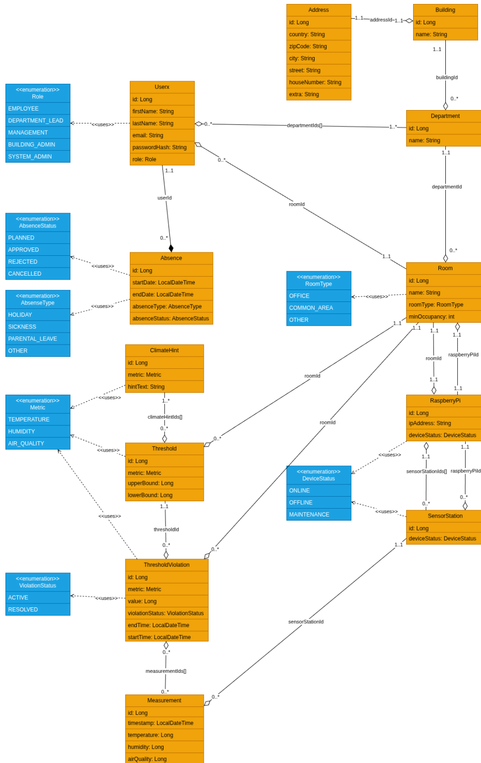
Abbildung 3: Class diagram V1
