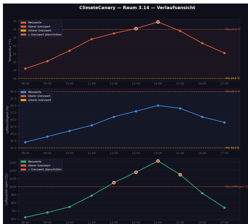
Abbildung 3: GUI Prototyp – Verlaufsansicht mit Grenzwert-Referenzlinien
