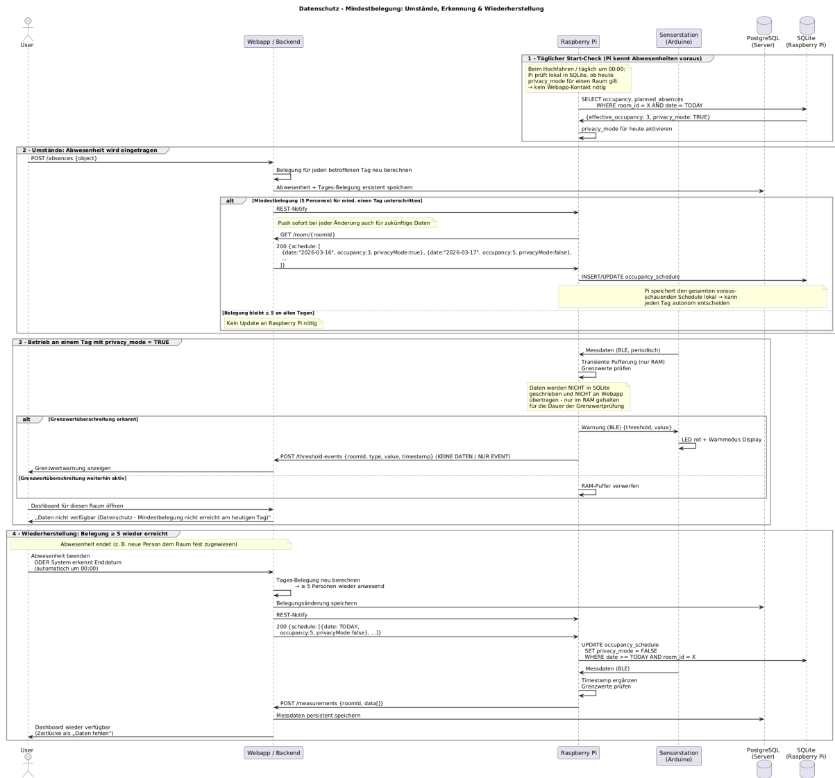
Abbildung 8: Sequenzdiagramm – Belegungs-Mindestgrenze
