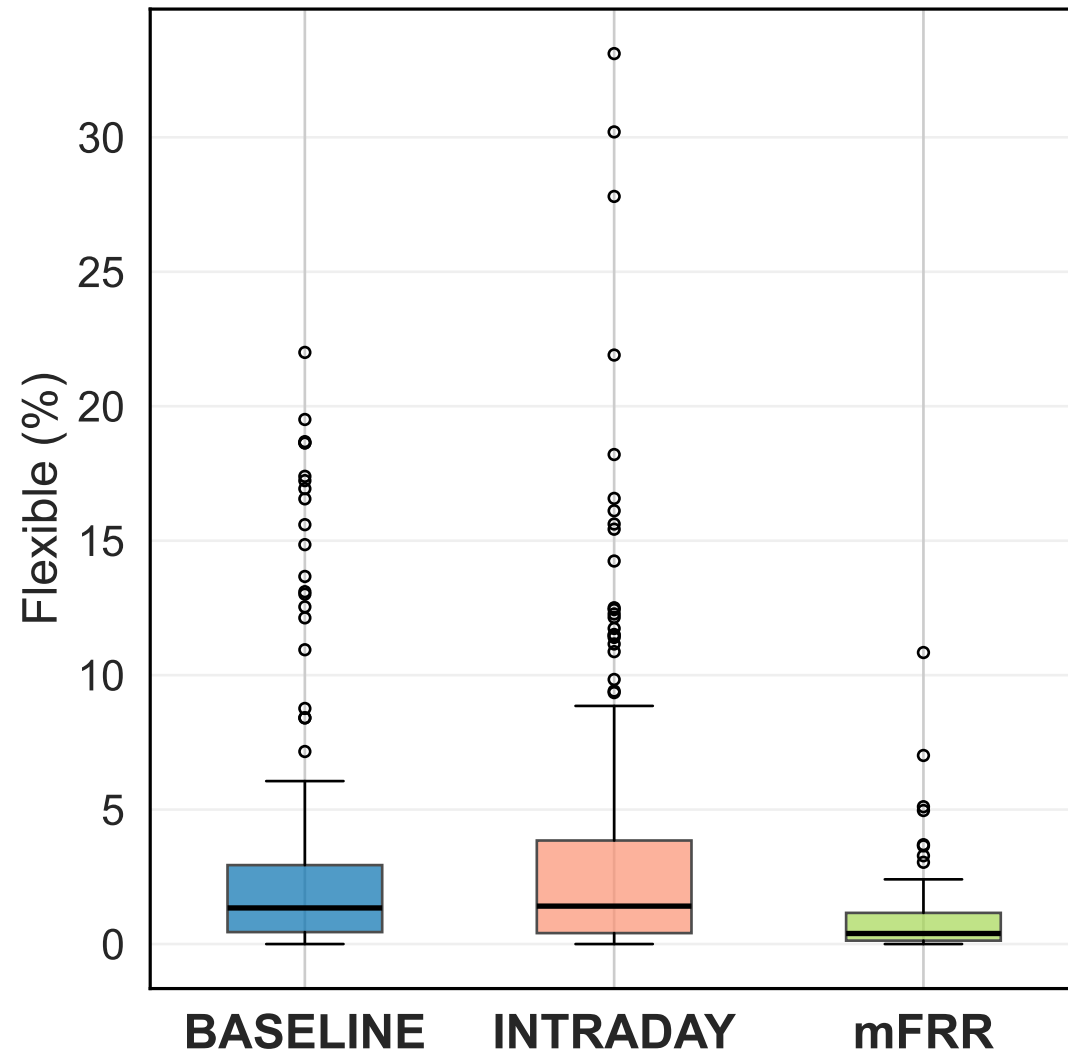
Flexible %
