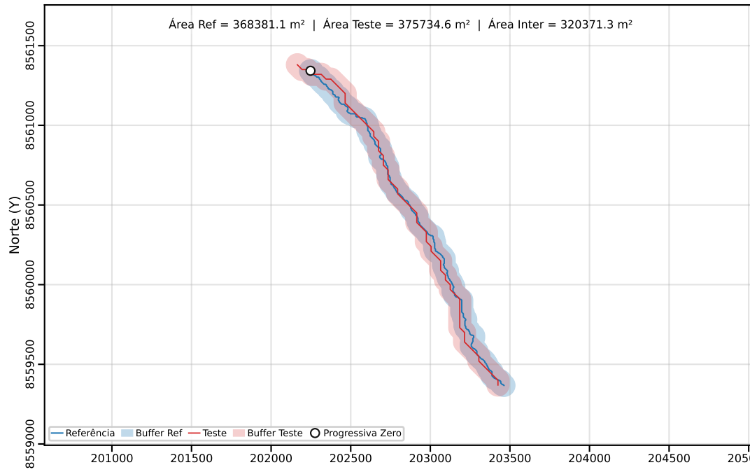
Classe C | PEC-PCD (Horizontal)=200.00 m | dm = 27.60
