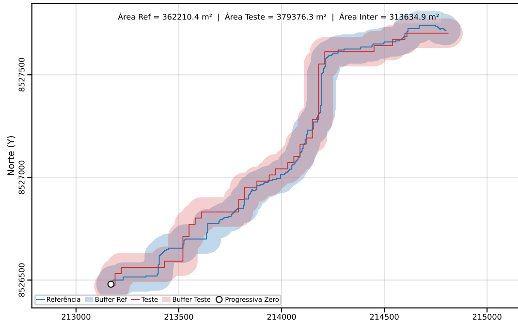
Classe C | PEC-PCD (Horizontal)=200.00 m | dm = 22.38
