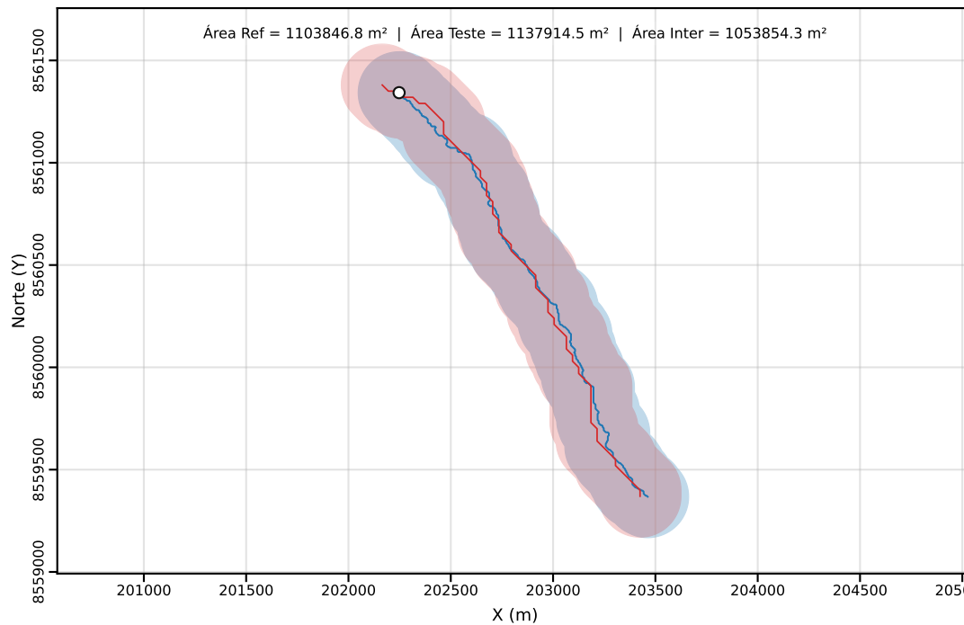
Classe C | PEC-PCD (Horizontal)=200.00 m | dm = 27.60
