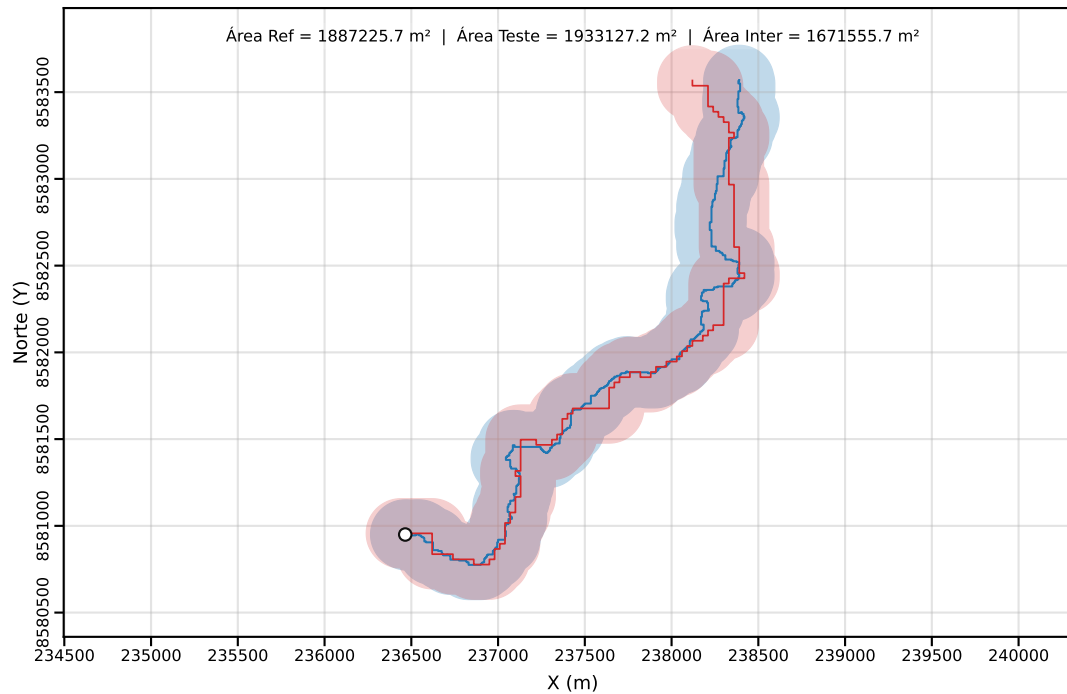
Classe C | PEC-PCD (Horizontal)=200.00 m | dm = 70.10
