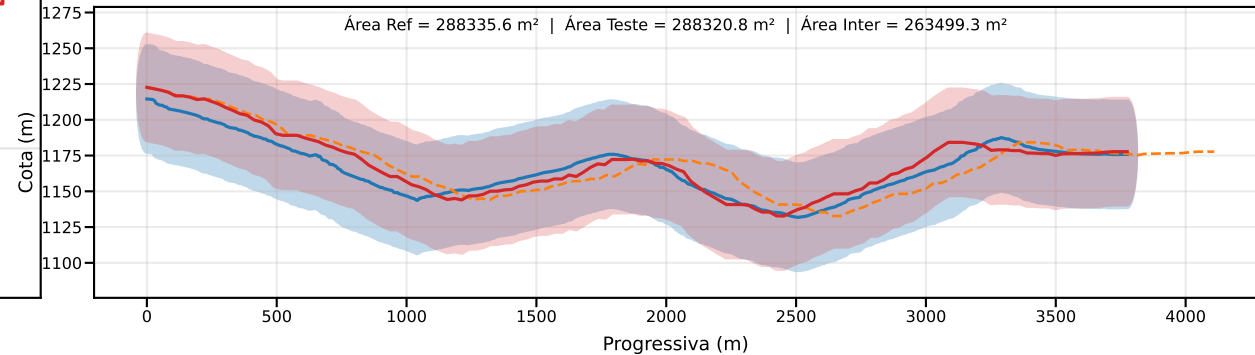
Classe D | PEC-PCD (Vertical)=37.5 m | EQ = 50m | dm = 10.15
