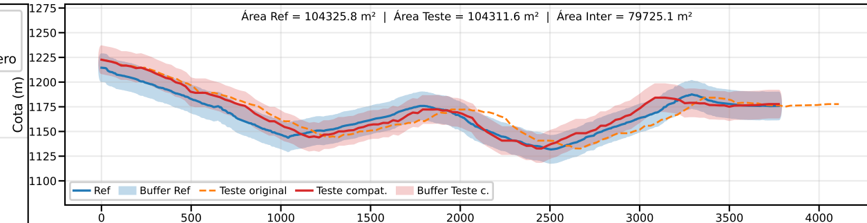
Classe B | PEC-PCD (Vertical)=25.0 m | EQ = 50m | dm = 10.15
