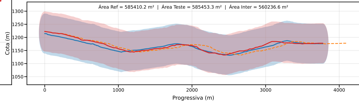
Classe D | PEC-PCD (Vertical)=75.0 m | EQ = 100m | dm = 10.13
