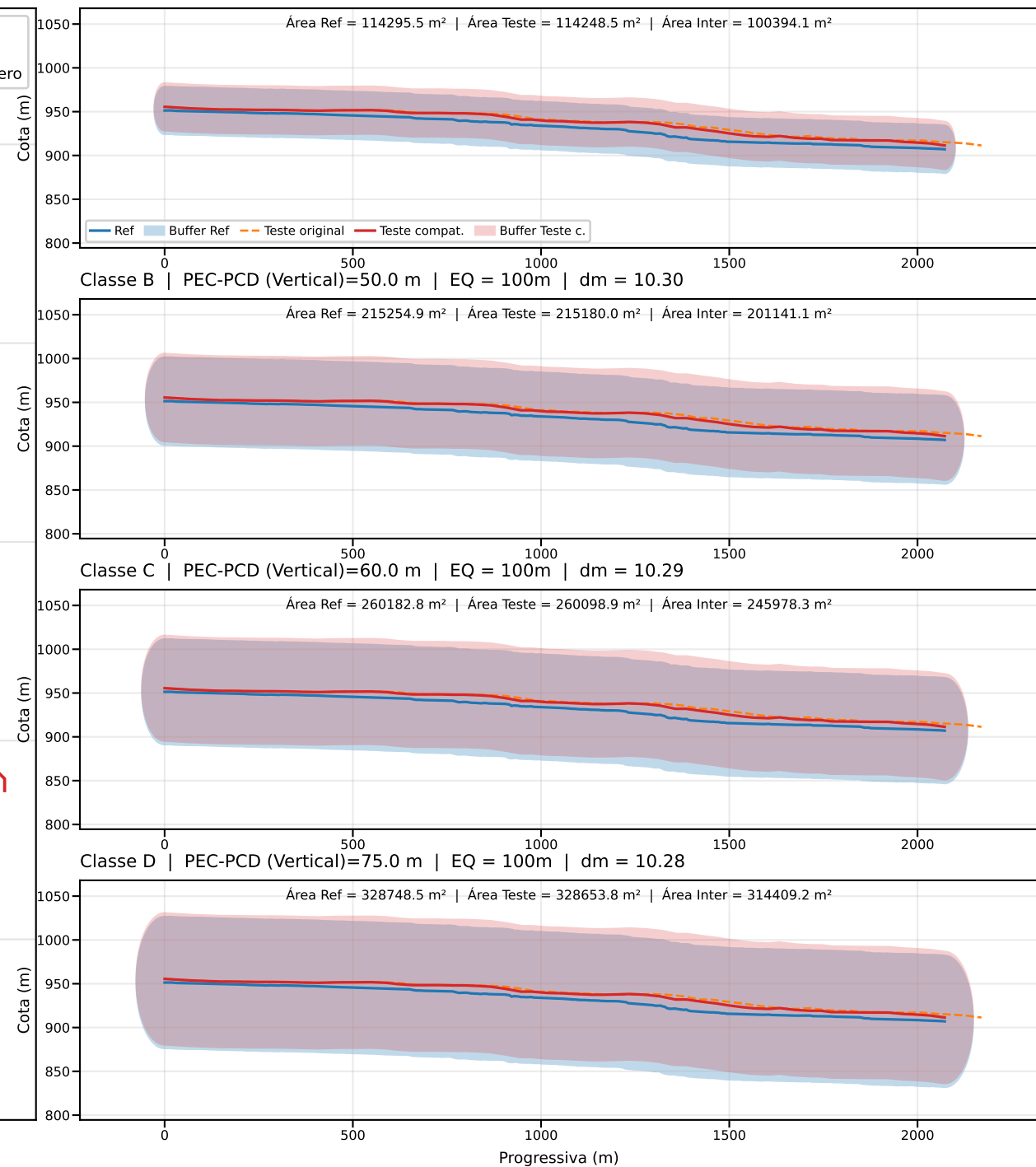
Classe A | PEC-PCD (Vertical)=27.0 m | EQ = 100m | dm = 10.32
