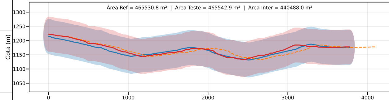
Classe D | PEC-PCD (Vertical)=75.0 m | EQ = 100m | dm = 10.13
