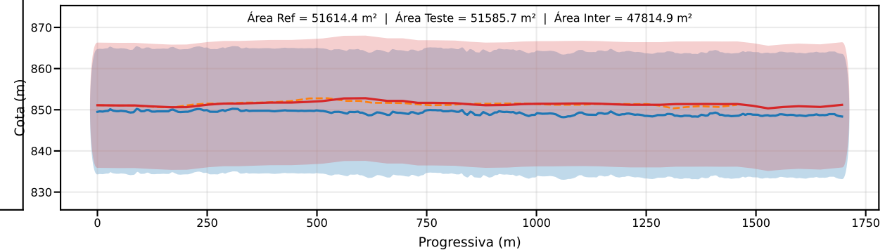
Classe D | PEC-PCD (Vertical)=15.0 m | EQ = 20m | dm = 3.47
