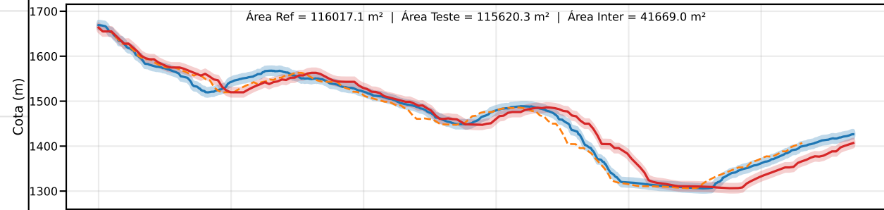
Classe C | PEC-PCD (Vertical)=12.0 m | EQ = 20m | dm = 22.53
