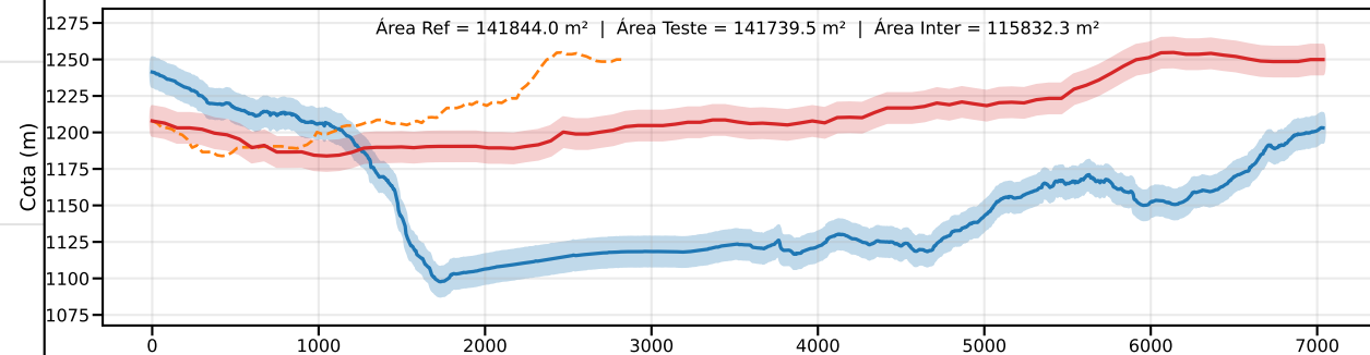
Classe C | PEC-PCD (Vertical)=12.0 m | EQ = 20m | dm = 5.77
