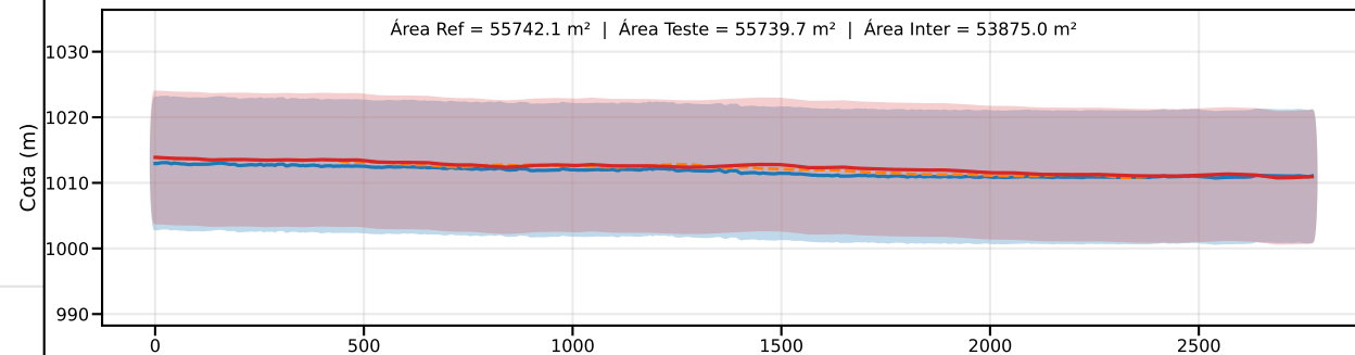
Classe C | PEC-PCD (Vertical)=12.0 m | EQ = 20m | dm = 1.05
