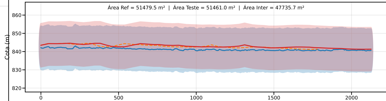
Classe D | PEC-PCD (Vertical)=15.0 m | EQ = 20m | dm = 2.74
