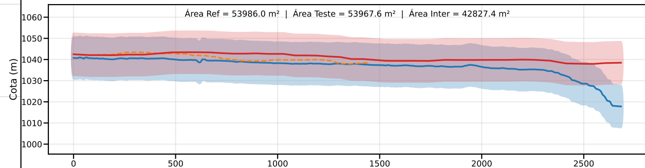
Classe C | PEC-PCD (Vertical)=12.0 m | EQ = 20m | dm = 6.55
