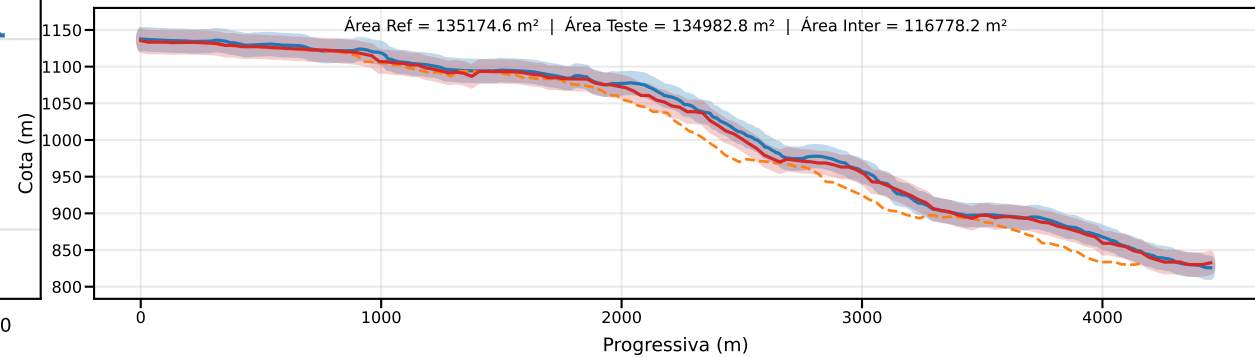
Classe D | PEC-PCD (Vertical)=15.0 m | EQ = 20m | dm = 6.42
