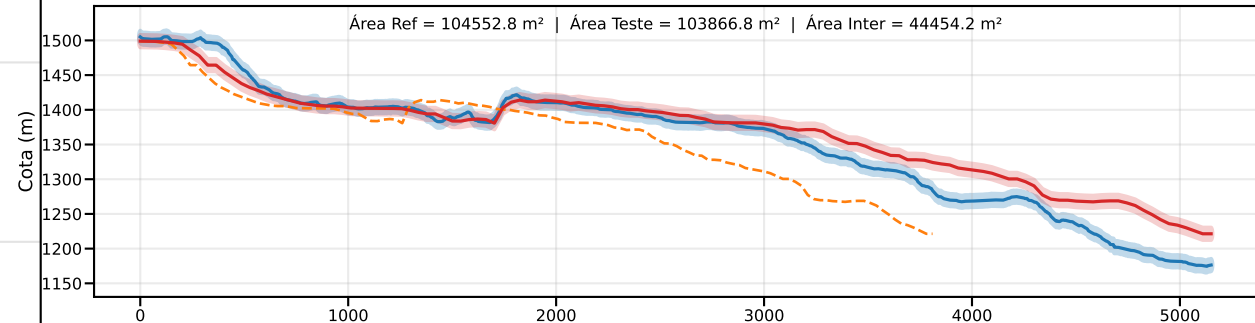
Classe C | PEC-PCD (Vertical)=12.0 m | EQ = 20m | dm = 20.64
