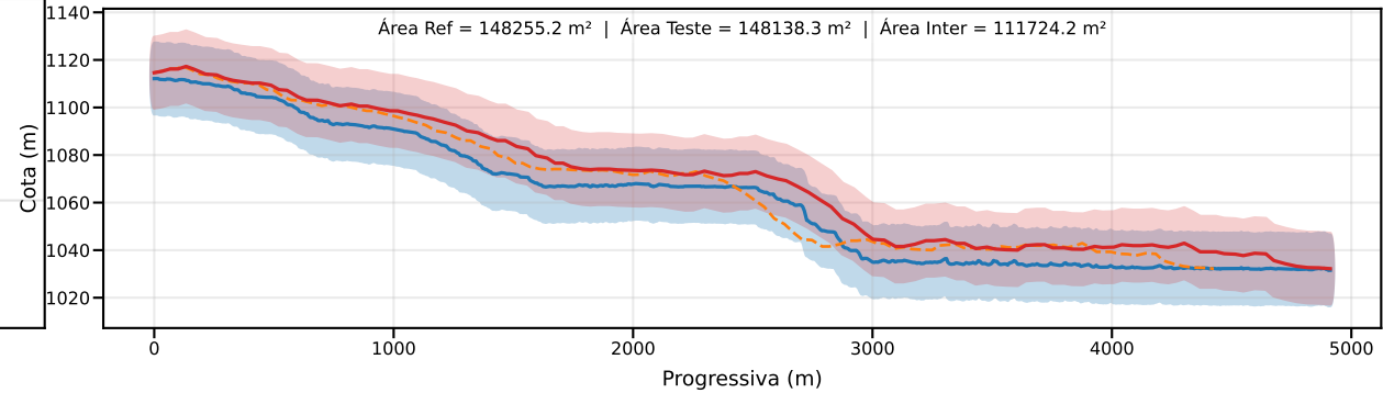
Classe D | PEC-PCD (Vertical)=15.0 m | EQ = 20m | dm = 11.62
