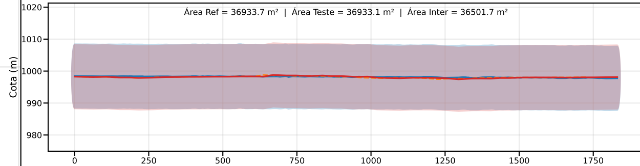
Classe C | PEC-PCD (Vertical)=12.0 m | EQ = 20m | dm = 0.37
