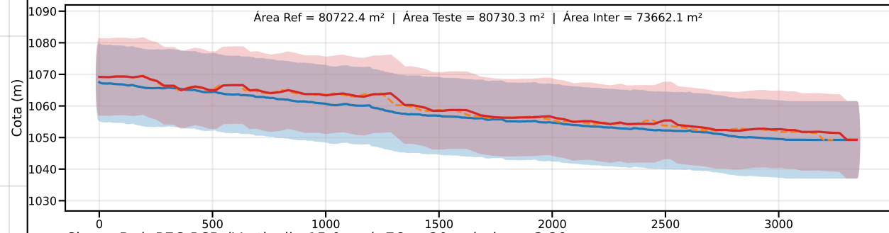
Classe D | PEC-PCD (Vertical)=15.0 m | EQ = 20m | dm = 3.29
