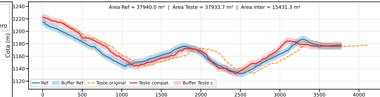
Classe B | PEC-PCD (Vertical)=10.0 m | EQ = 20m | dm = 10.15
