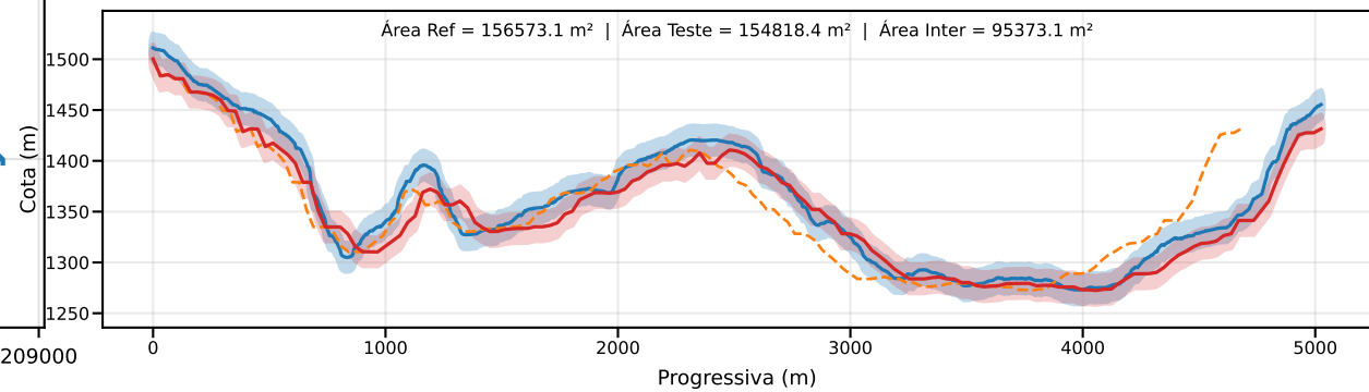
Classe D | PEC-PCD (Vertical)=15.0 m | EQ = 20m | dm = 18.63
