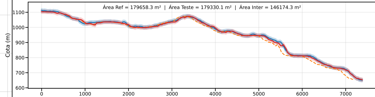
Classe D | PEC-PCD (Vertical)=15.0 m | EQ = 20m | dm = 7.05
