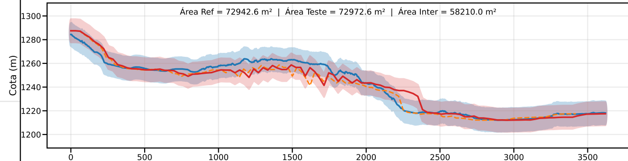
Classe C | PEC-PCD (Vertical)=12.0 m | EQ = 20m | dm = 6.34
