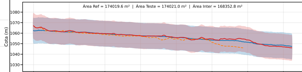
Classe D | PEC-PCD (Vertical)=15.0 m | EQ = 20m | dm = 1.23
