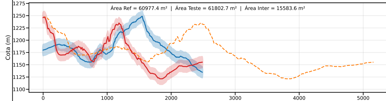
Classe D | PEC-PCD (Vertical)=15.0 m | EQ = 20m | dm = 31.41
