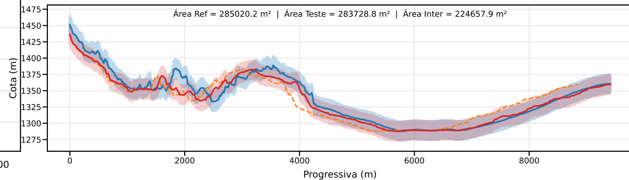
Classe D | PEC-PCD (Vertical)=15.0 m | EQ = 20m | dm = 10.03
