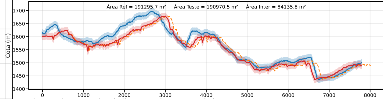
Classe D | PEC-PCD (Vertical)=15.0 m | EQ = 20m | dm = 23.54
