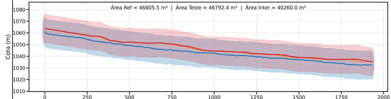
Classe D | PEC-PCD (Vertical)=15.0 m | EQ = 20m | dm = 5.28
