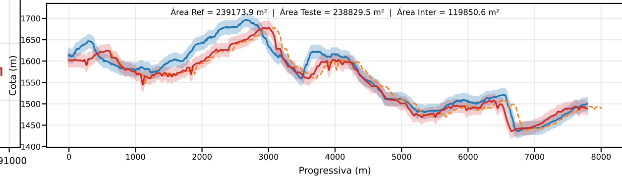
Classe D | PEC-PCD (Vertical)=15.0 m | EQ = 20m | dm = 23.54
