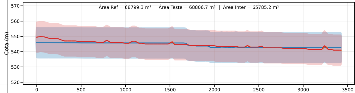
Classe C | PEC-PCD (Vertical)=12.0 m | EQ = 20m | dm = 1.38
