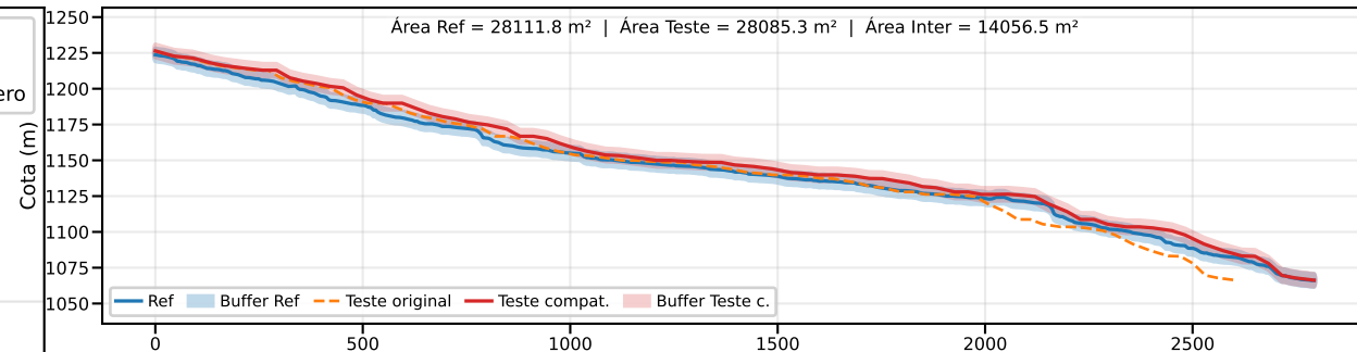
Classe B | PEC-PCD (Vertical)=10.0 m | EQ = 20m | dm = 7.87
