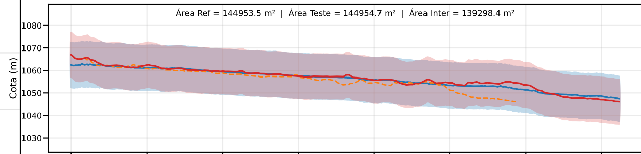
Classe C | PEC-PCD (Vertical)=12.0 m | EQ = 20m | dm = 1.23
