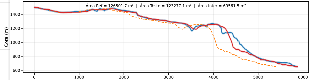
Classe C | PEC-PCD (Vertical)=12.0 m | EQ = 20m | dm = 15.71
