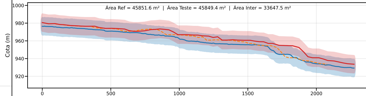
Classe C | PEC-PCD (Vertical)=12.0 m | EQ = 20m | dm = 8.36
