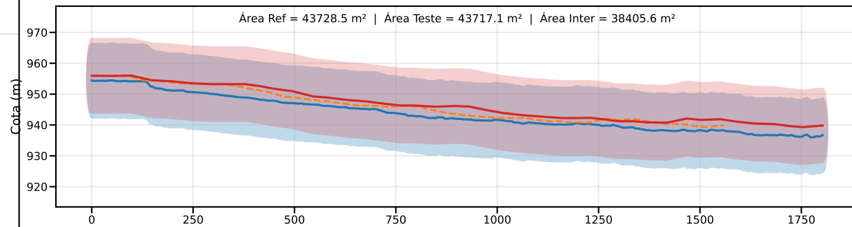
Classe D | PEC-PCD (Vertical)=15.0 m | EQ = 20m | dm = 4.59
