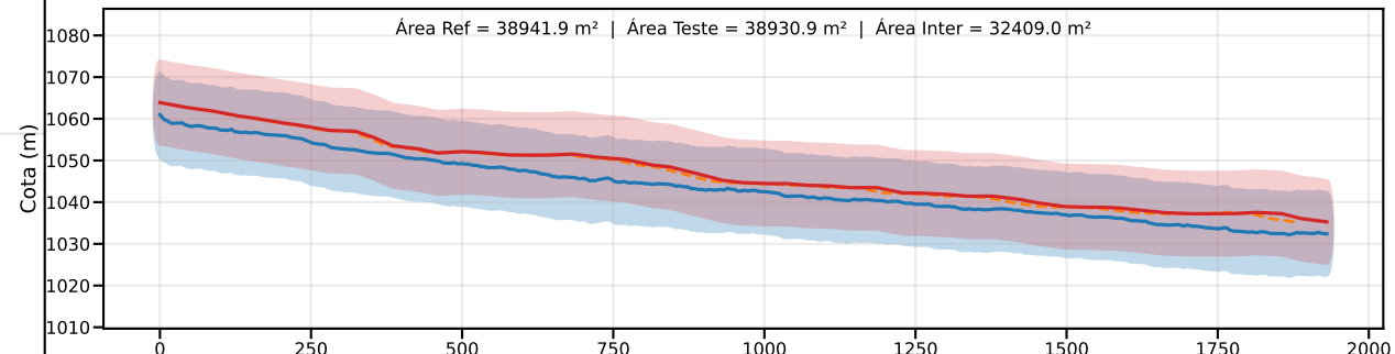
Classe C | PEC-PCD (Vertical)=12.0 m | EQ = 20m | dm = 5.27
