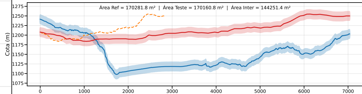
Classe D | PEC-PCD (Vertical)=15.0 m | EQ = 20m | dm = 5.77
