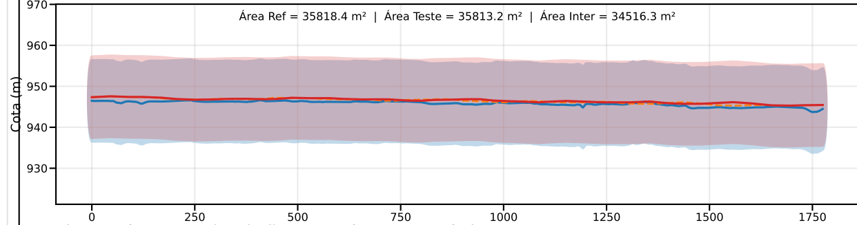
Classe C | PEC-PCD (Vertical)=12.0 m | EQ = 20m | dm = 1.14
