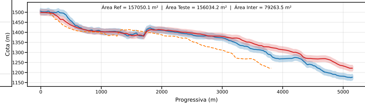
Classe D | PEC-PCD (Vertical)=15.0 m | EQ = 20m | dm = 23.49
