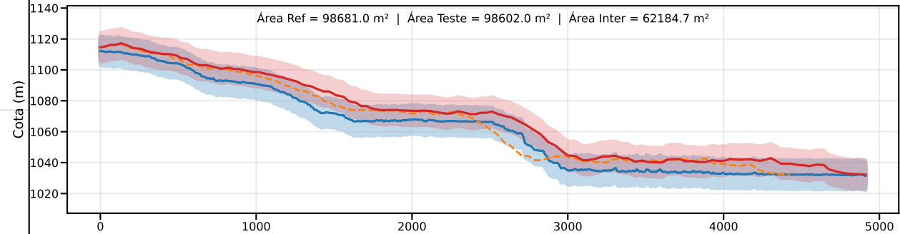
Classe C | PEC-PCD (Vertical)=12.0 m | EQ = 20m | dm = 11.63
