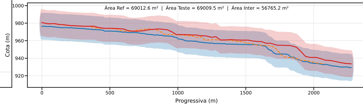
Classe D | PEC-PCD (Vertical)=15.0 m | EQ = 20m | dm = 8.36
