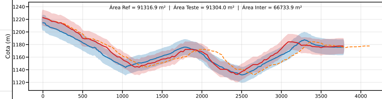
Classe D | PEC-PCD (Vertical)=15.0 m | EQ = 20m | dm = 10.15
