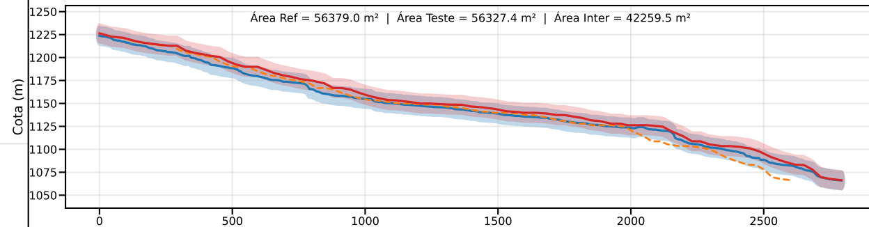
Classe C | PEC-PCD (Vertical)=12.0 m | EQ = 20m | dm = 7.87
