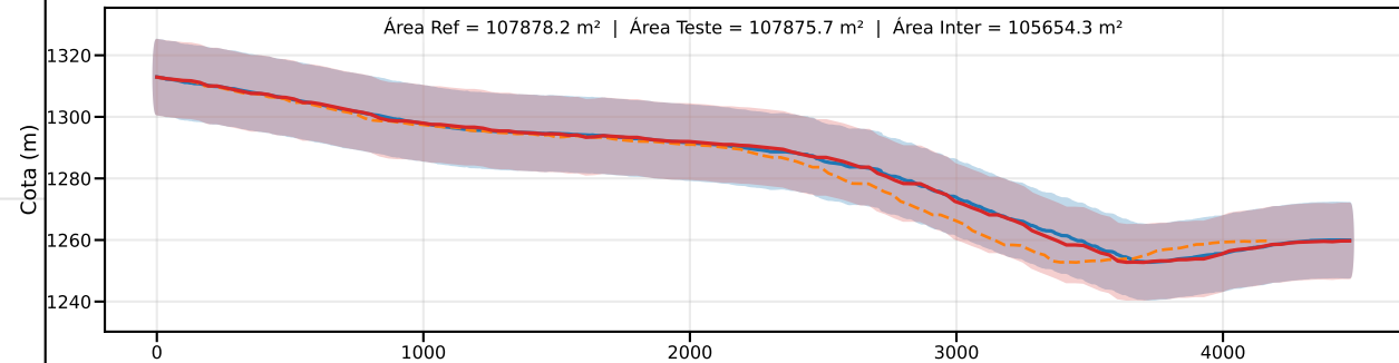
Classe D | PEC-PCD (Vertical)=15.0 m | EQ = 20m | dm = 0.78
