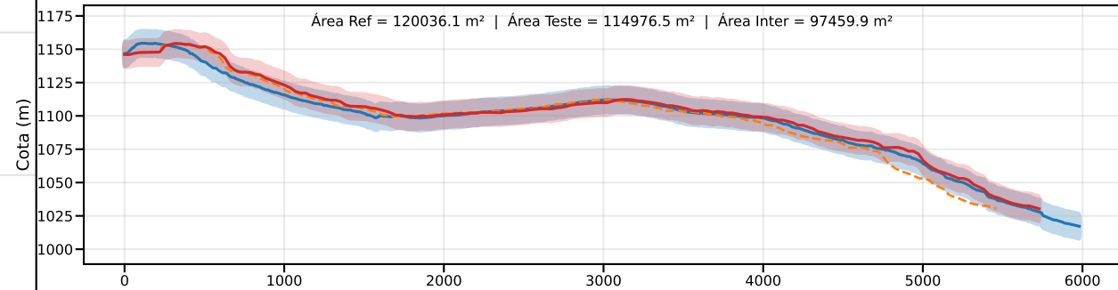
Classe C | PEC-PCD (Vertical)=12.0 m | EQ = 20m | dm = 6.44
