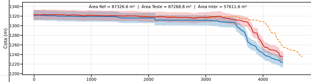
Classe C | PEC-PCD (Vertical)=12.0 m | EQ = 20m | dm = 11.14
