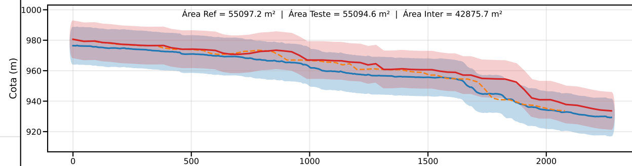
Classe D | PEC-PCD (Vertical)=15.0 m | EQ = 20m | dm = 8.36
